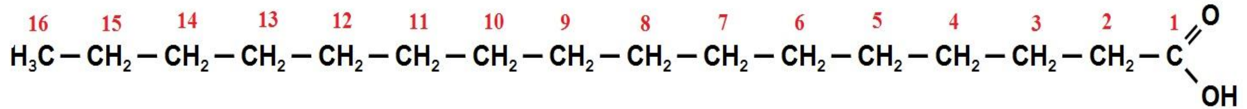
Пальмитиновая кислота (C 16 )
