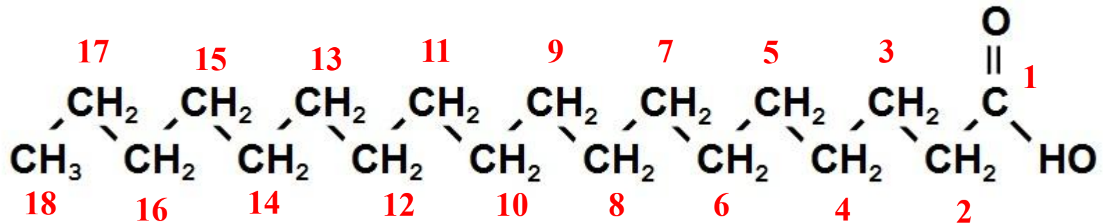
Пальмитиновая кислота (C 16 )
