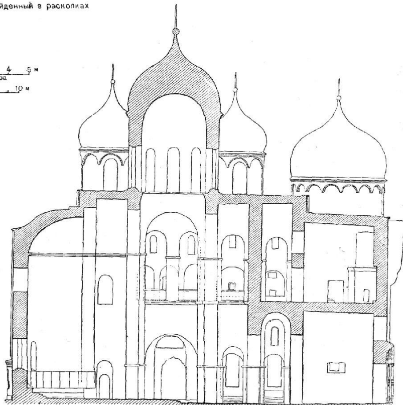
Продольный разрез
