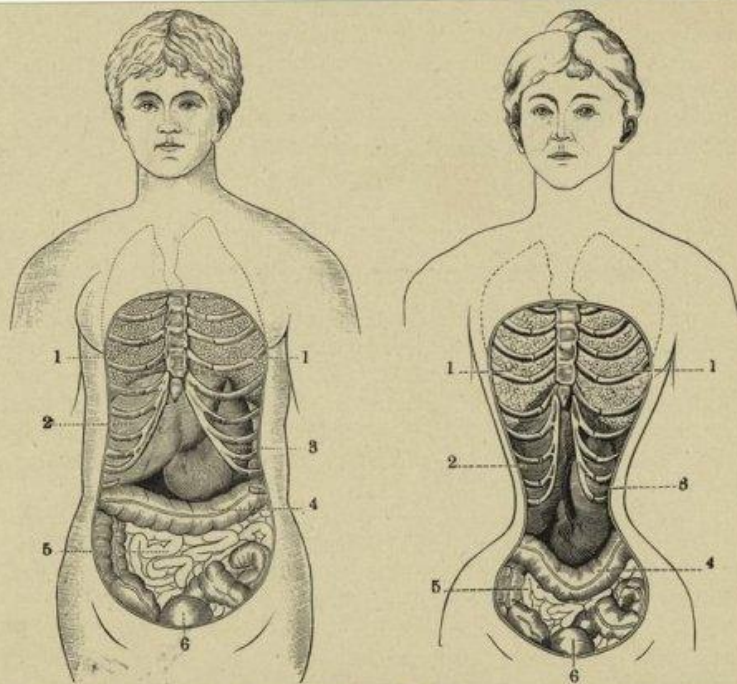
Fig. 69. Natürliche Lage der Bauchorgane. Fig. 70. Vershobene Lage der Bauchorgane. 1 Lunge. 2 Leber. 3 Magen. 4 Dickdarm. 5 Dünndarm. 6 Blase.
