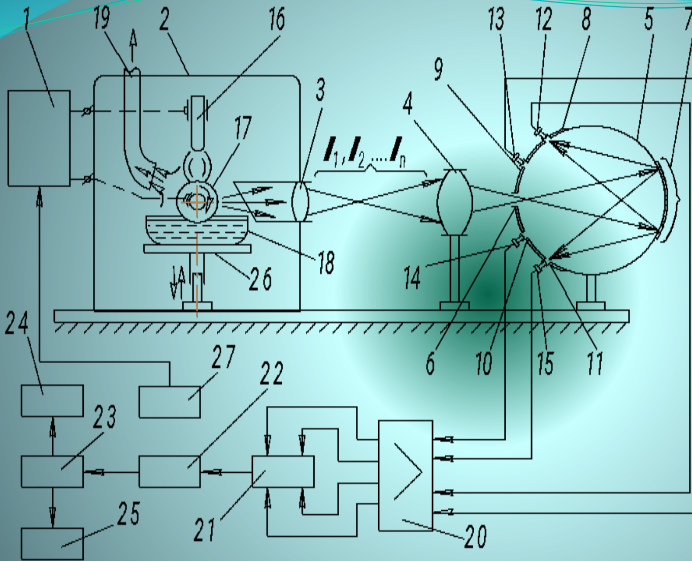
Структурная схема и блок-схема атомно-эмиссионной установки типа МФС-7
