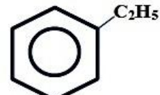
этилбензол
