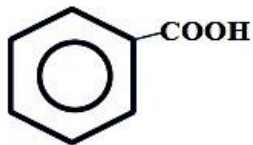
бензолкарбоновая к-та (бензойная)
