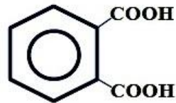
фталевая к-та (бензол-1,2-дикарбоновая)
