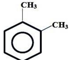
диметилбензол (ксилол)
