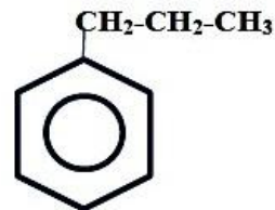
пропилбензол
