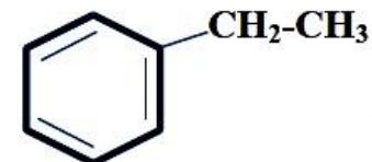
этилбензол
