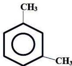
1,3-диметилбензол ( мета -ксилол)
