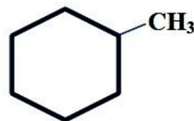
метилциклогексан
