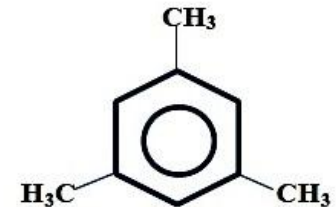
1,3,5-триметилбензол (мезитилен)
