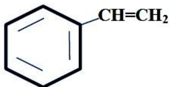
винилбензол (стирол)
