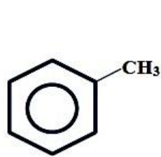
метилбензол (толуол)
