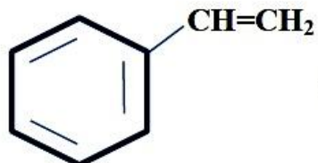
винилбензол (стирол)
