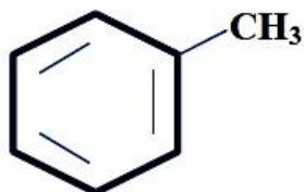
метилбензол (толуол)
