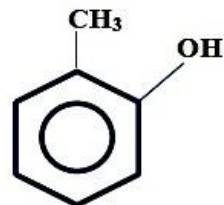
метилфенол (крезол)
