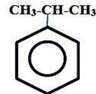
изопропилбензол (кумол)
