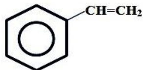
винилбензол (стирол)
