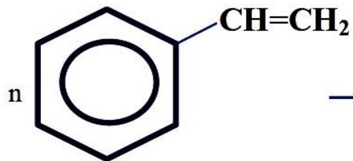
винилбензол (стирол)
