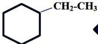
этилциклогексан
