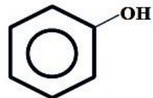
гидроксibenзол (фенол)
