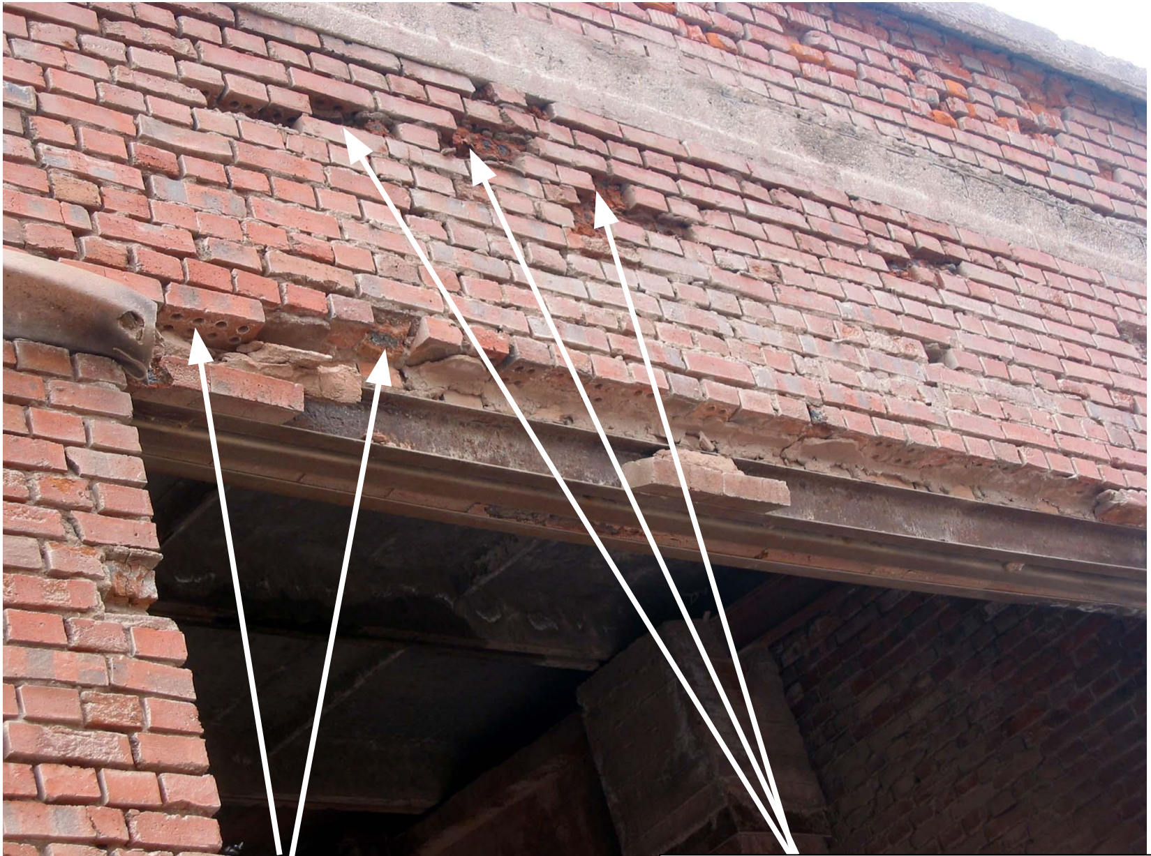
Эрозия отдельных кирпичей. Выпадение кирпичей из-за недостаточной длины площадки опирания
