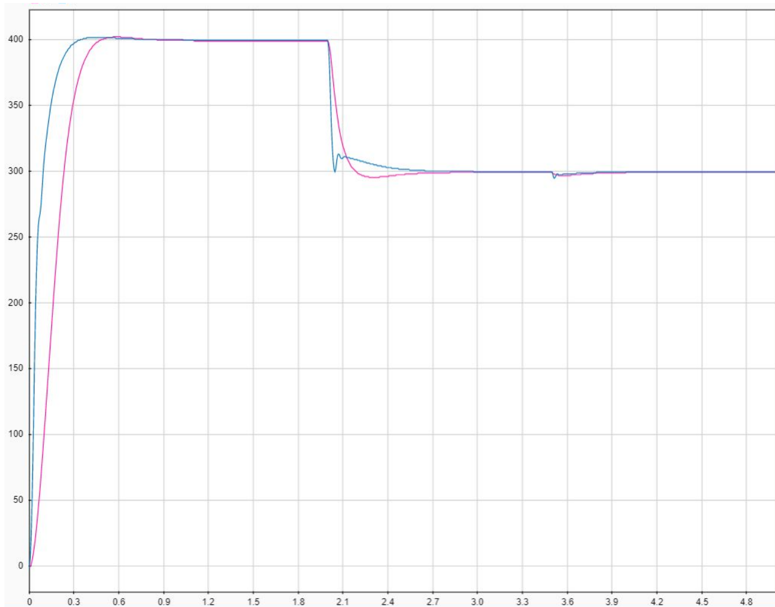
ПИД-регулятор
