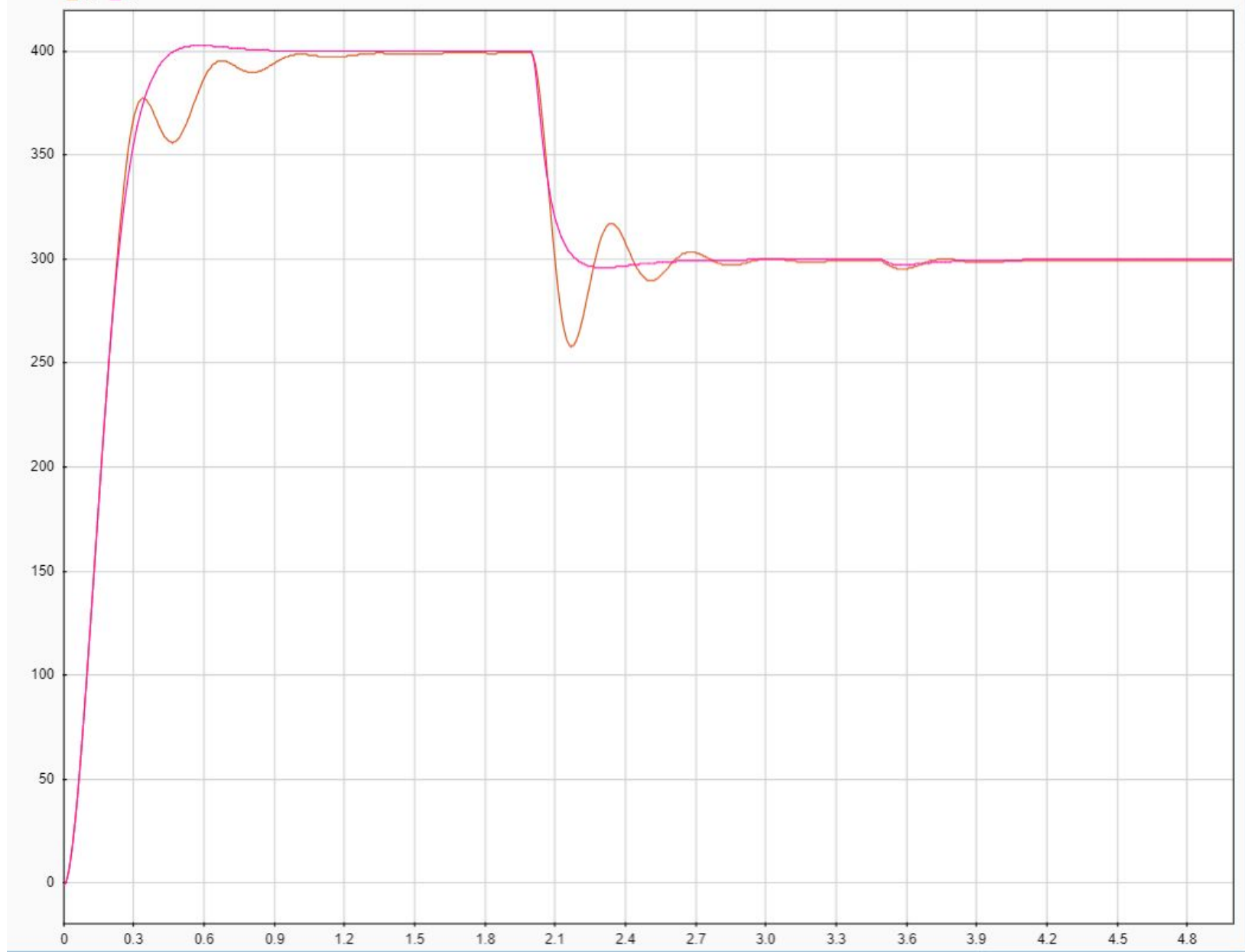
ПИД-регулятор
