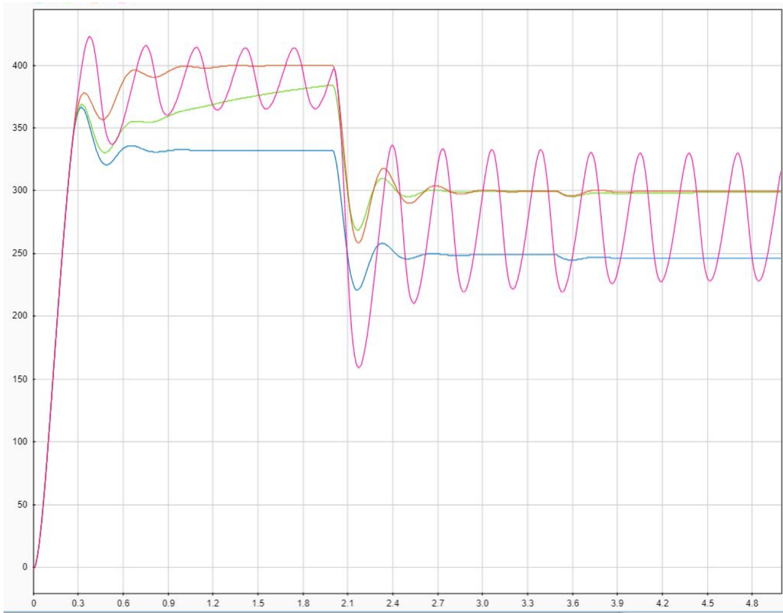
ПИ-регулятор
