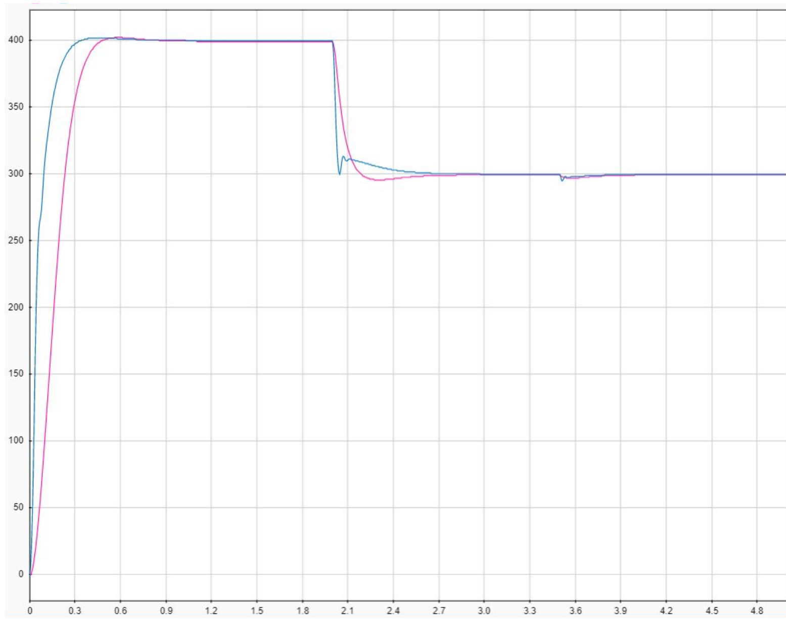
ПИД-регулятор
