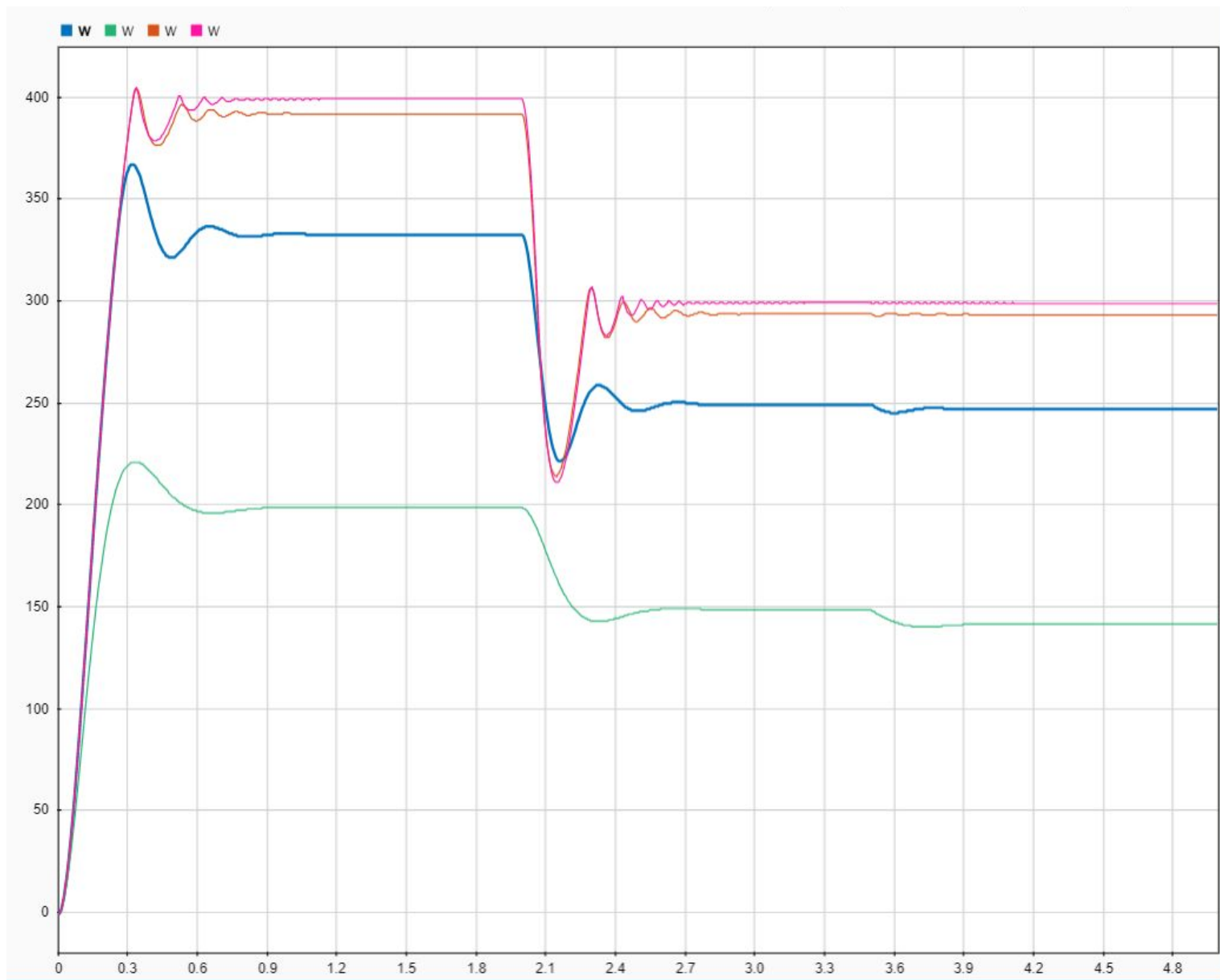
П-регулятор
