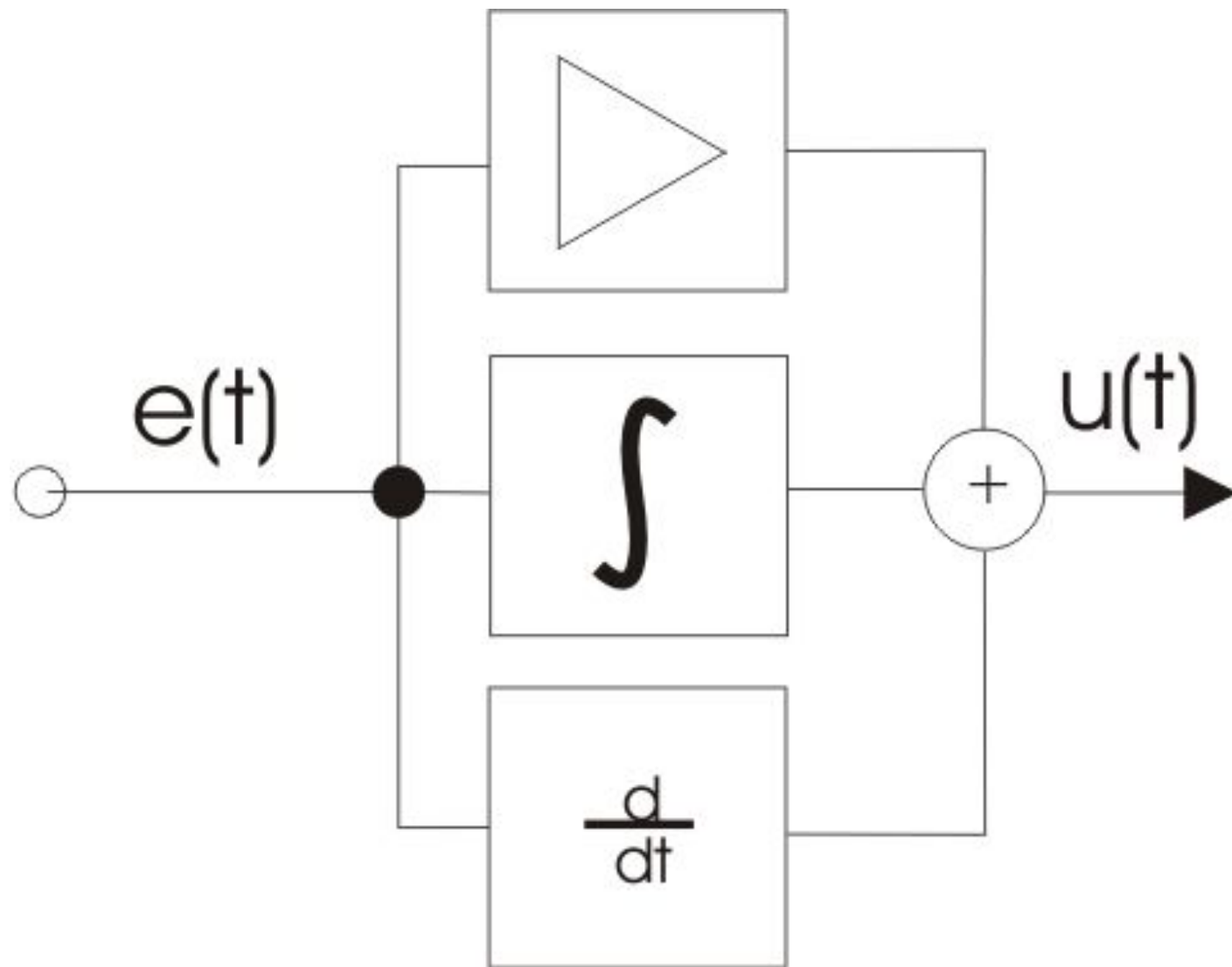
ПИД-регулятор
