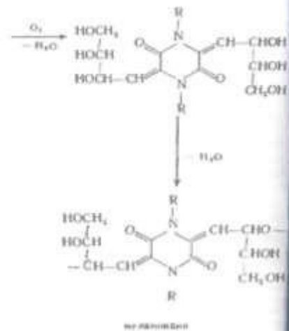
Схема образования меланоидина (в задние — карамель)
