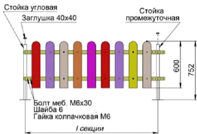
Рисунок 1 – Внешний вид ограждения секционного. Основные размеры. Монтаж
