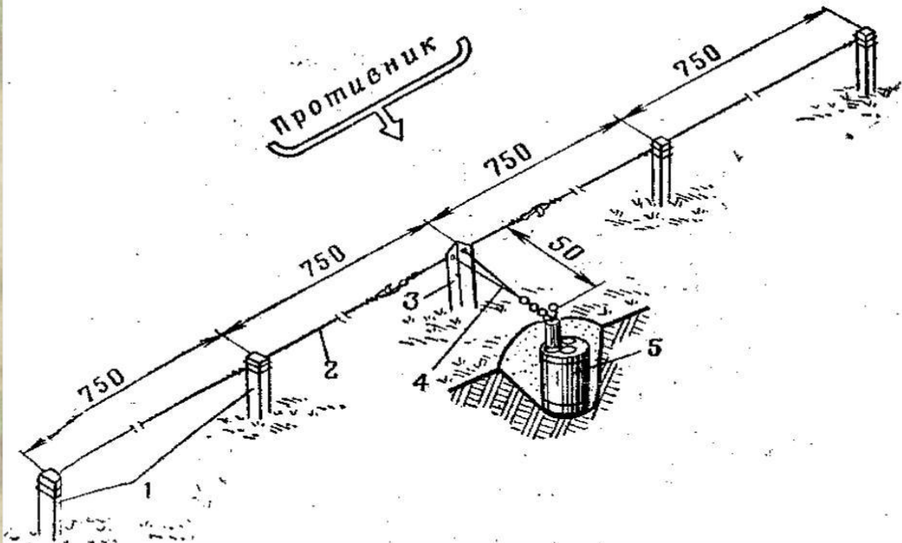
Схема установки мины ОЗМ-
