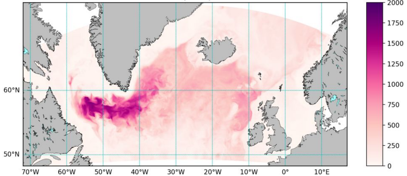
Mixed layer depth
