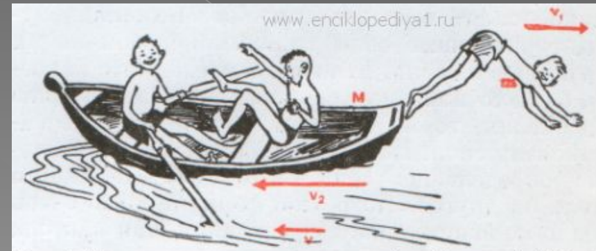
Рис. 4. По закону о сохранении движения (m+M)v= mv_1+Mv_2 .
