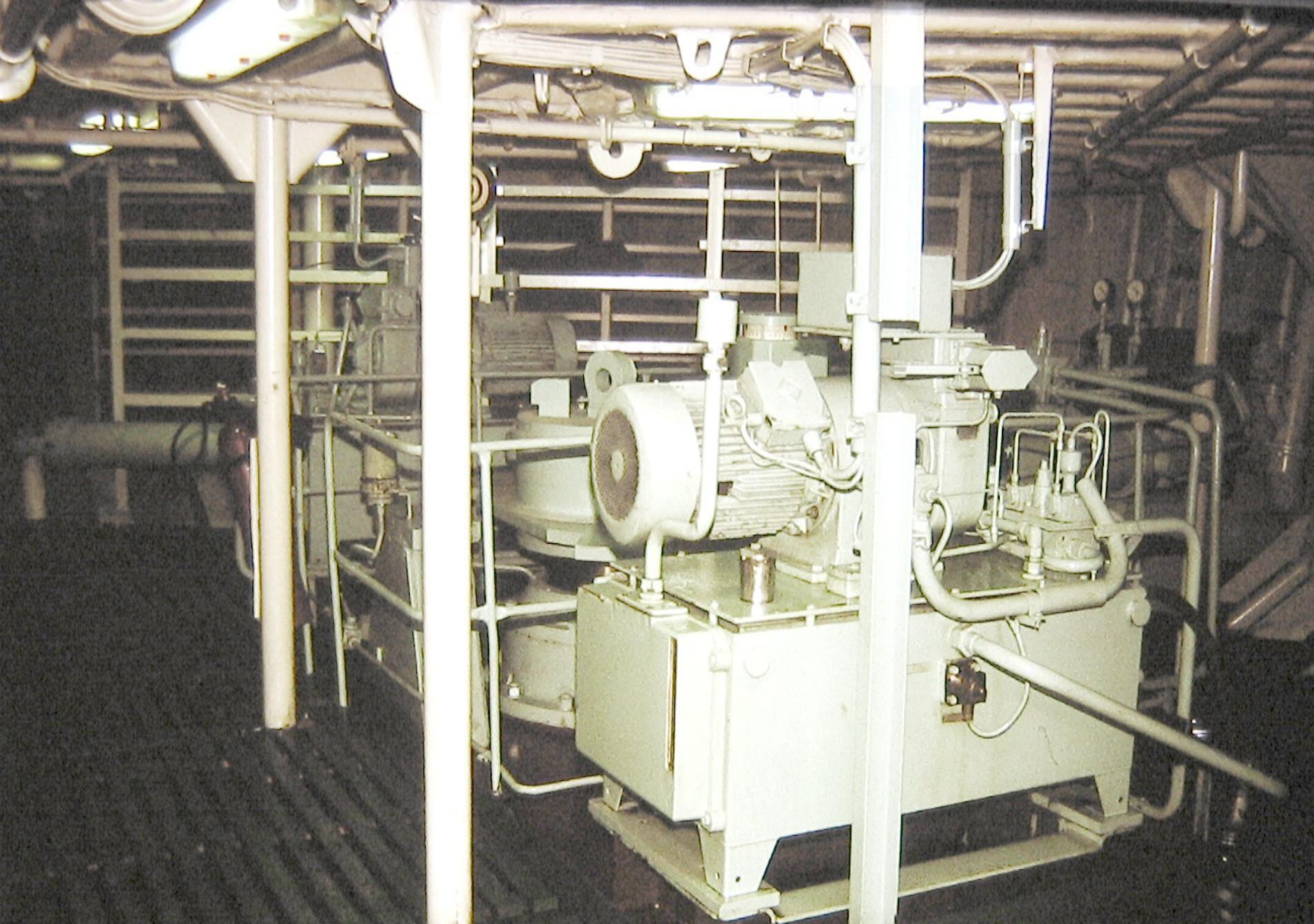
румпельное отделение
