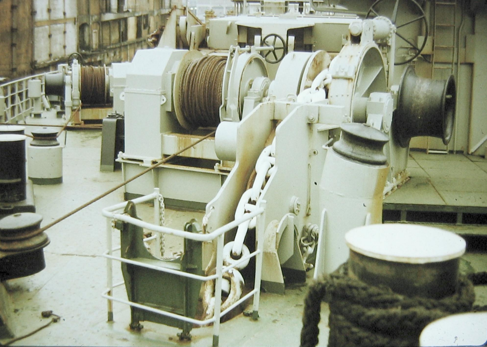
автоматическая швартовная лебедка и полубрашпиль
