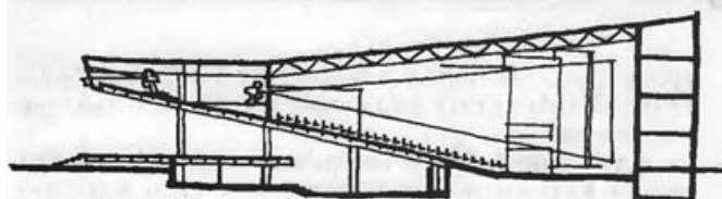
Кинотеатр «Первомайский» на 93/20. Архитекторы Д. Солопов 1969. Общий вид, схема разреза
