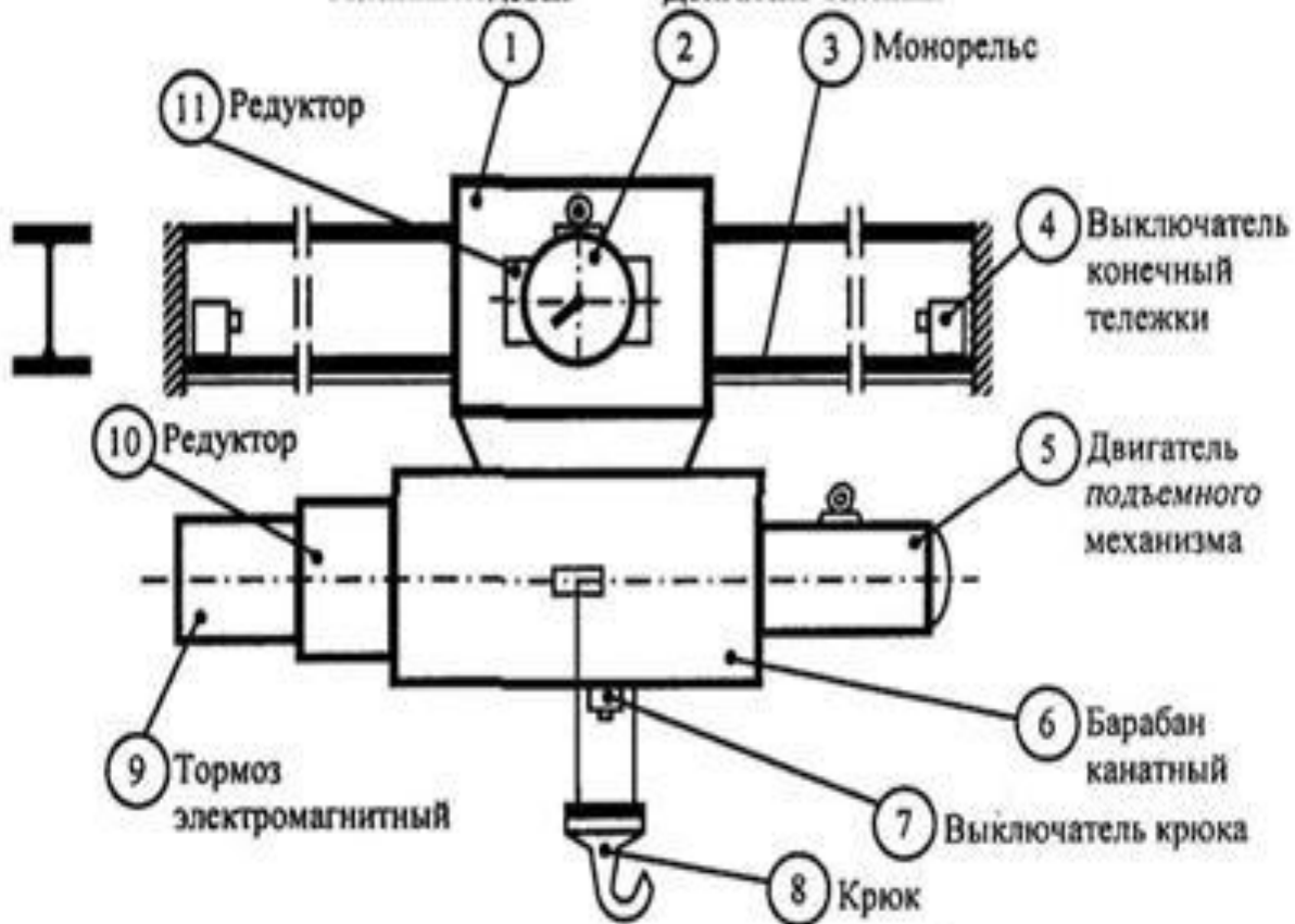
Тележка ходовая
