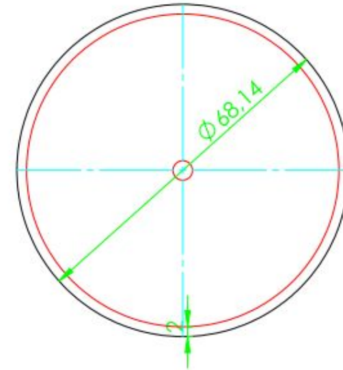
LID
