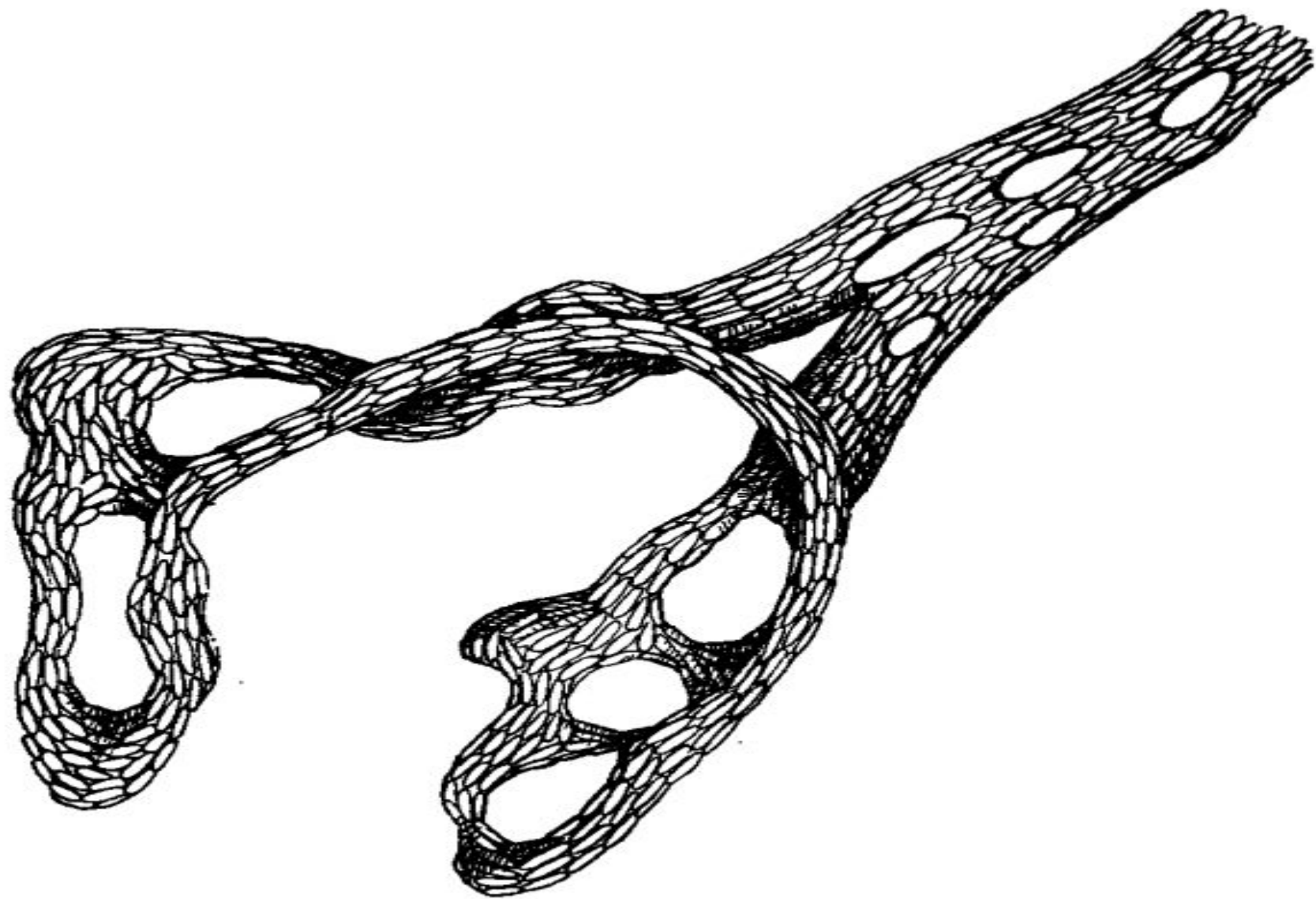
Рис. 68. Устройство ловчего приспособления хищной бактерии Tetrahobacter (по Перфильеву, Габе, 1961).
