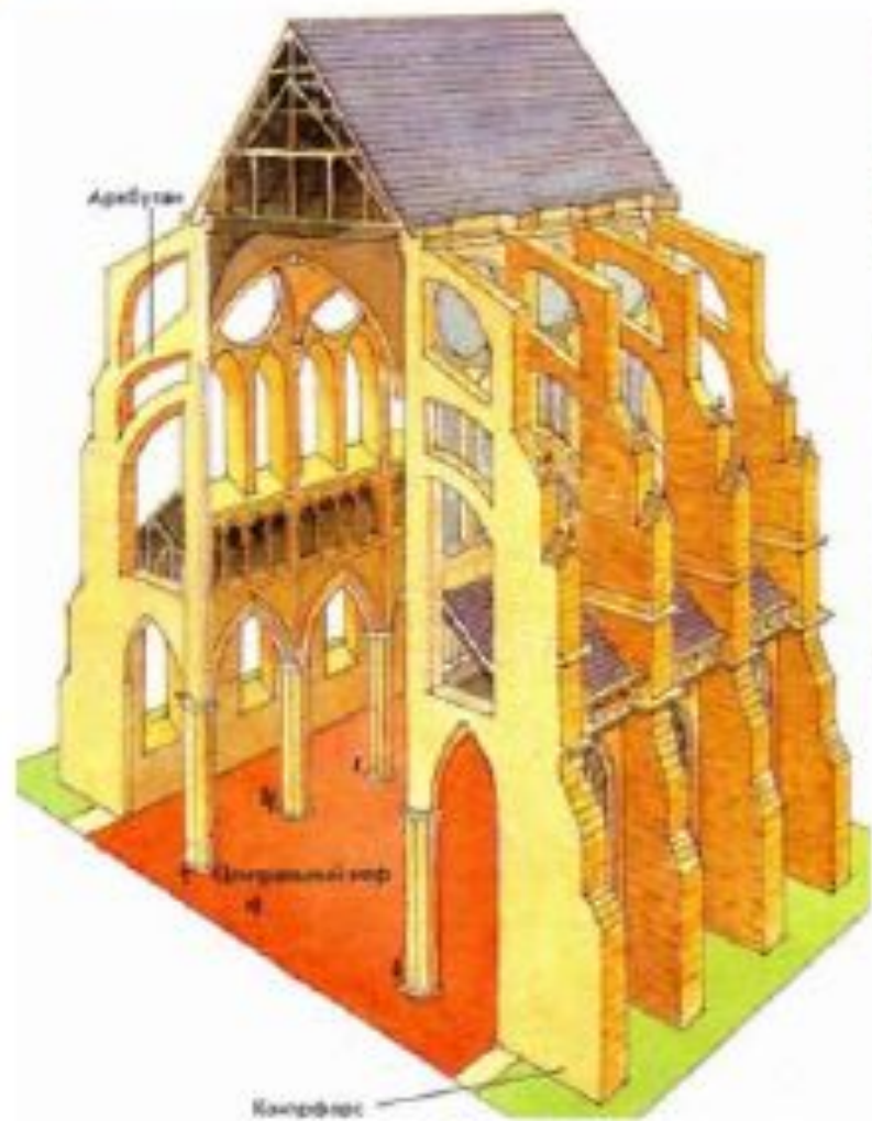
Каркасная система готического собора
