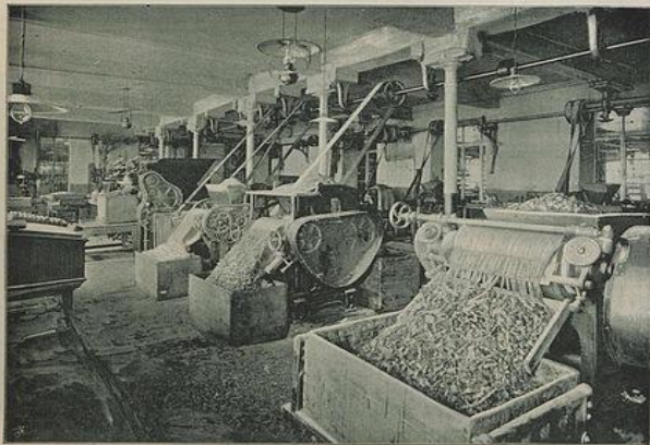
Стружечные машины. Авторства Э. Голца.
