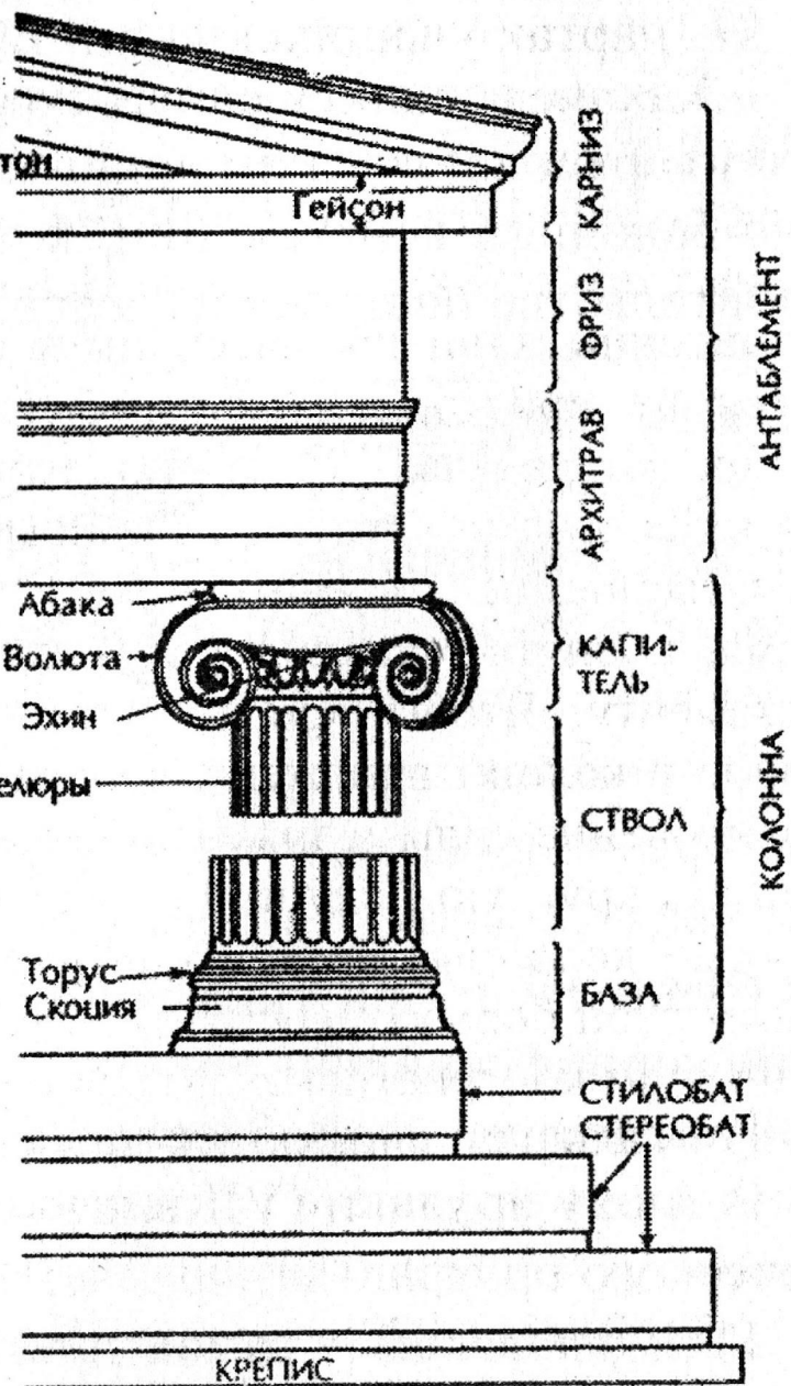
Схема ионического ордера
