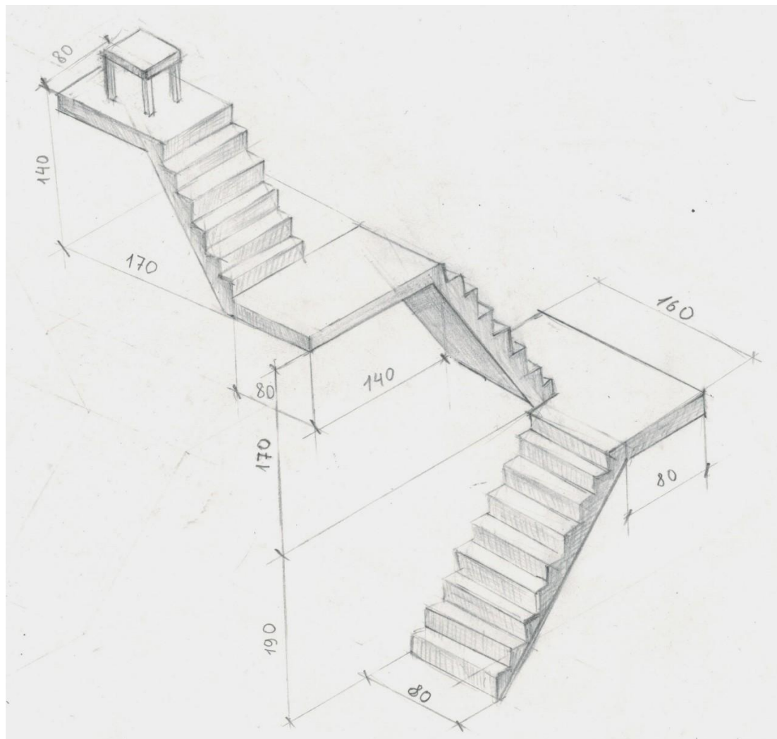
1. Закрученная лестница, имеющая на своем завершении смотровую площадку с посадочным местом
