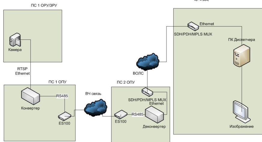
Структурная схема организации ТВН на ПС
