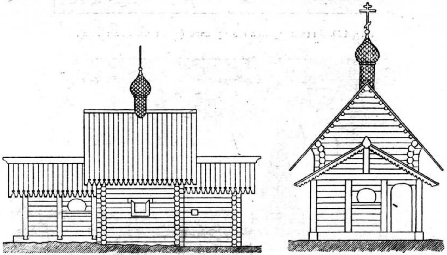
Рис. 122 и 123. Церковь преп. Лазаря въ Муромскомъ монастырѣ. Чертежи Л. Даля.
