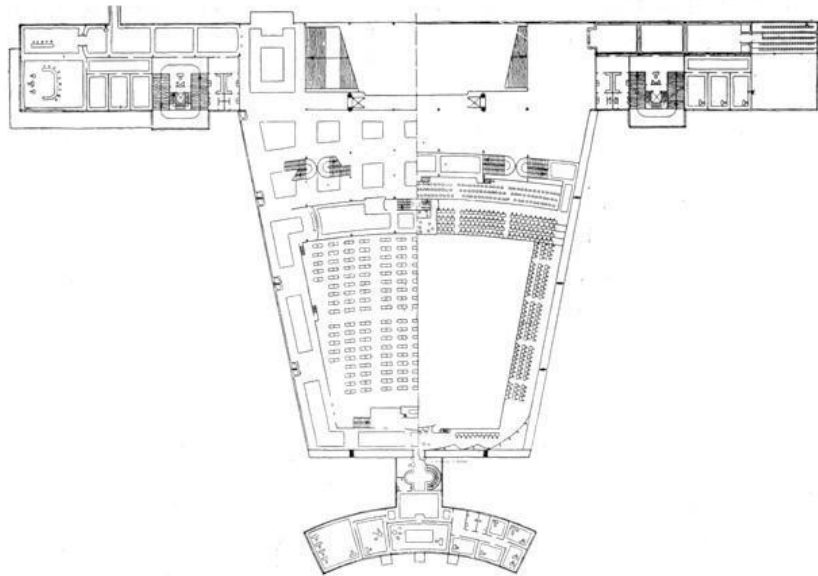
Проект Дворца Лиги Наций в Женеве, арх. Ле Корбюзье и П. Жанпере, 1927 г.
