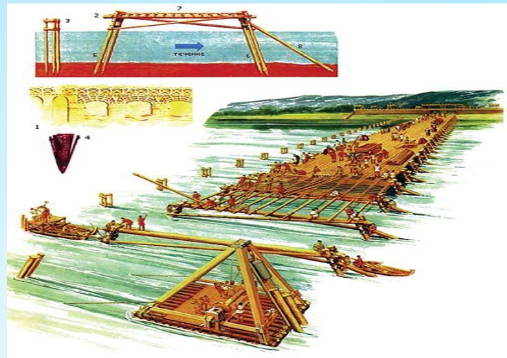
Қалқымалы көпір
