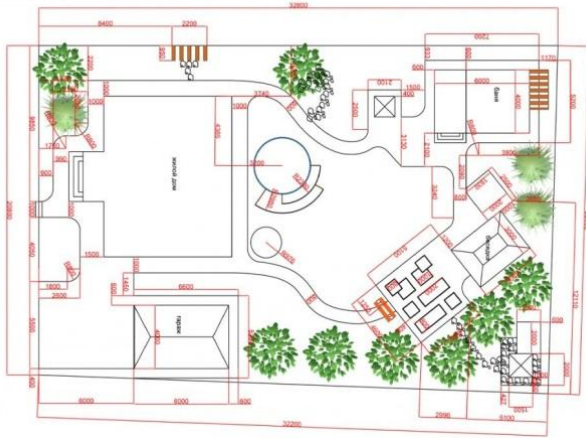
РАЗБИВОЧНЫЙ ЧЕРТЕЖ НА ПЛАНИРОВКУ М 1:200
