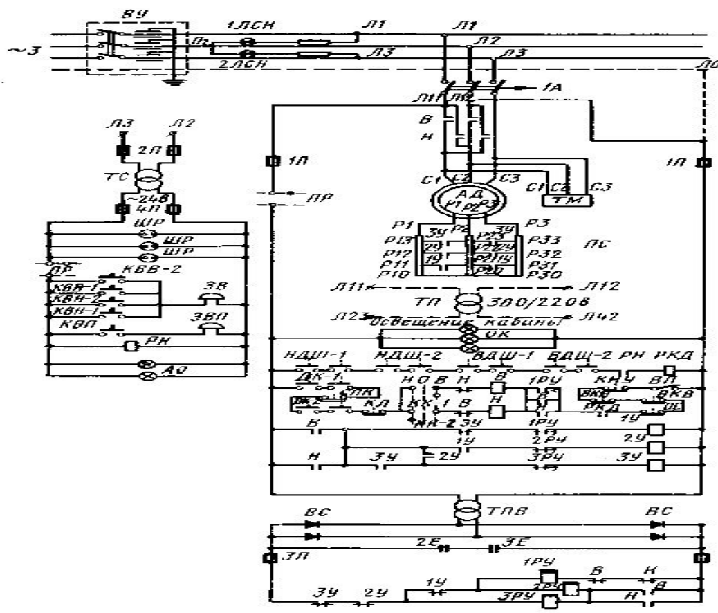
Рис. 93. Принципиальная электрическая схема грузового лифта с рычажным управлением на две остановки
