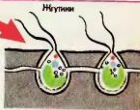
Клетки вольвокса
