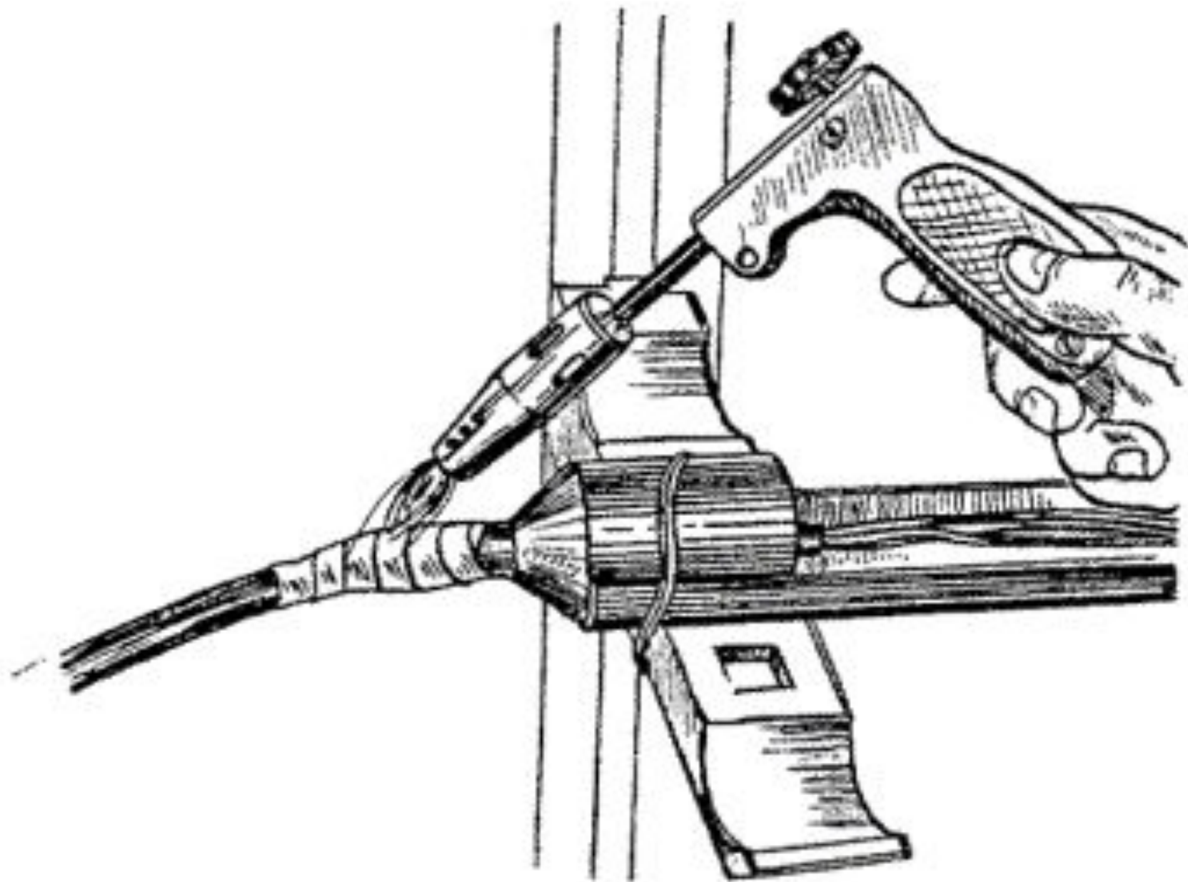
Приварка полиэтиленового конуса к кабелю
