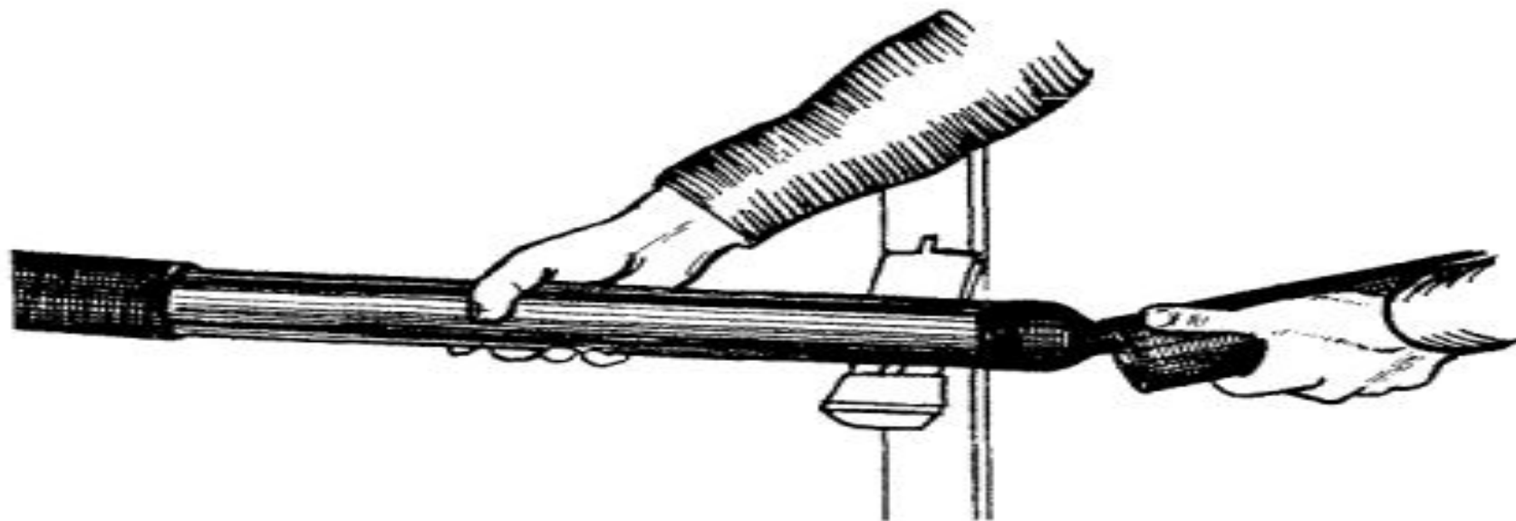
Установка цилиндрических частей полиэтиленовой муфты
