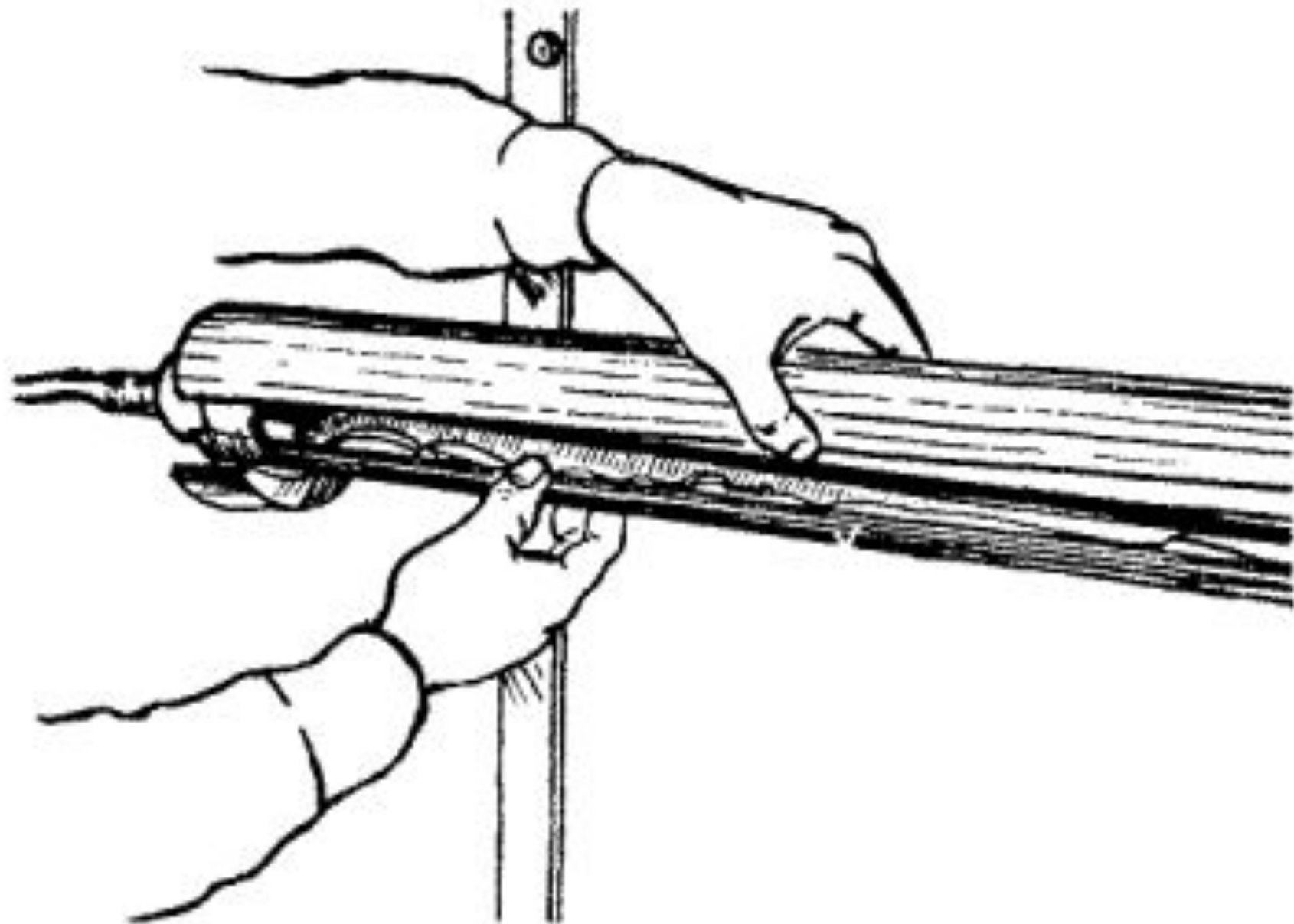
Установка второй части металлического каркаса
