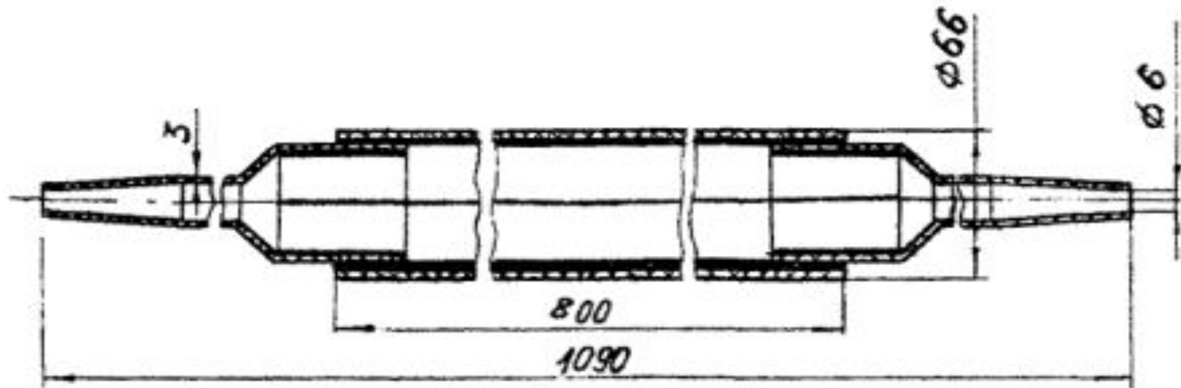
Соединительная муфта СМОК
