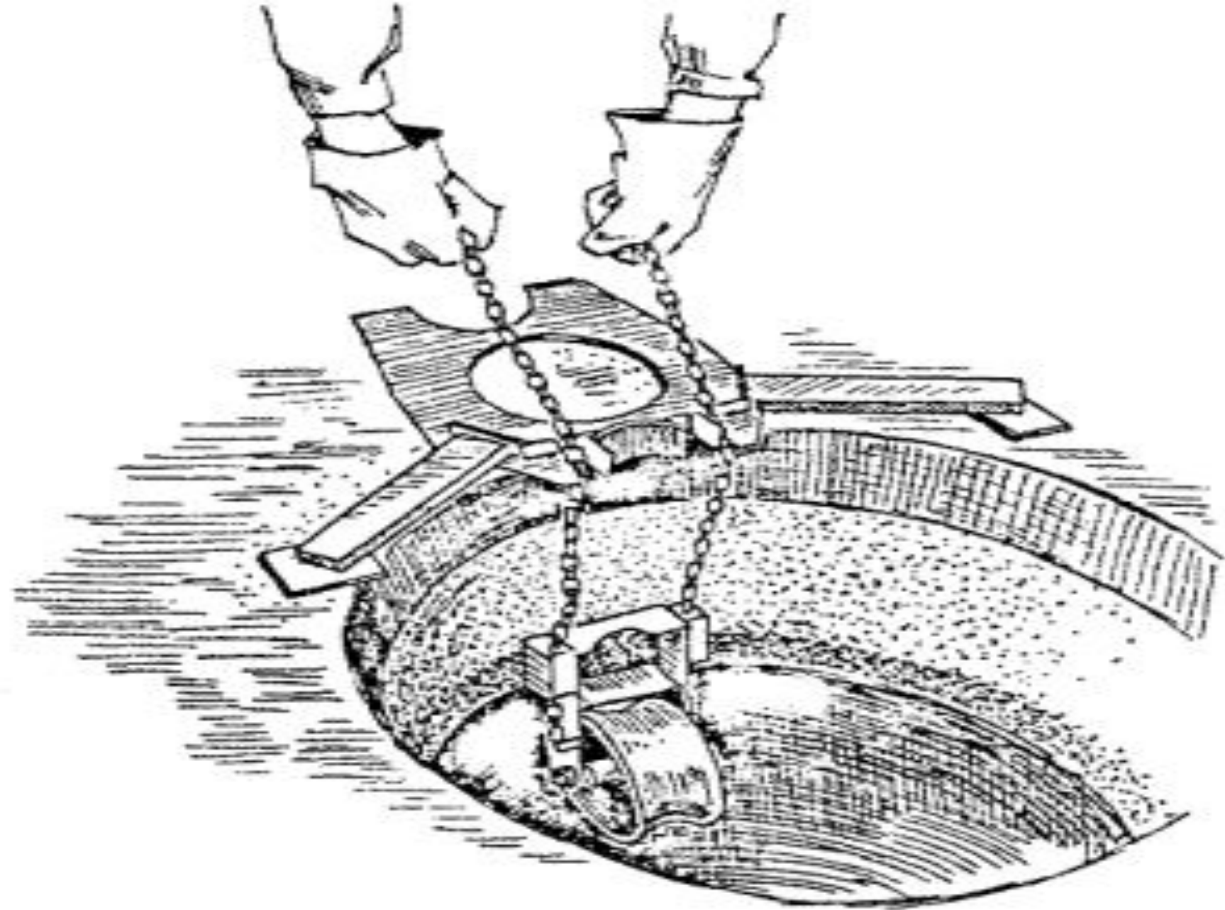
Установка люкоогибных роликов
