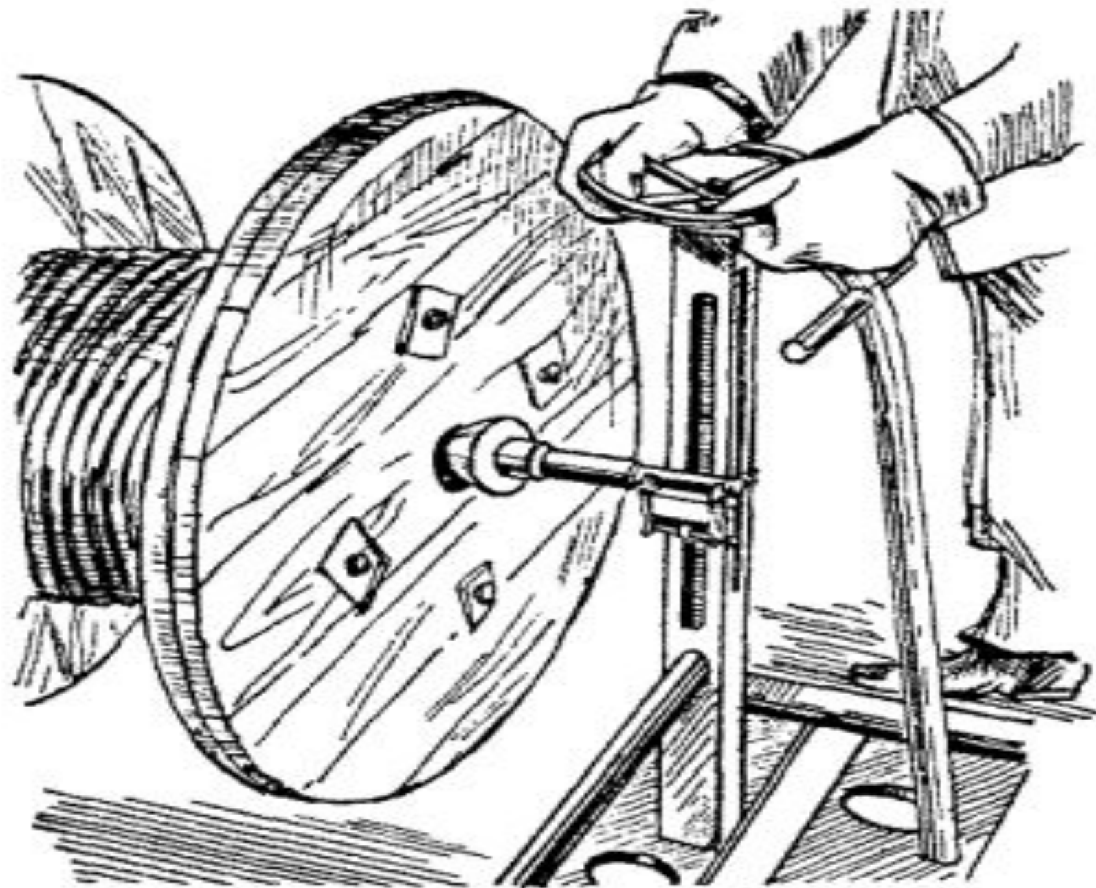
Устройство для размотки кабеля с барабана
