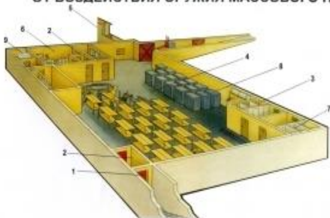
СХЕМА УБЕЖИЩА ДЛЯ ДЛИТЕЛЬНОЙ ЗАЩИТЫ ОТ ВОЗДЕЙСТВИЯ ОРУЖИЯ МАССОВОГО ПОРАЖЕНИЯ
