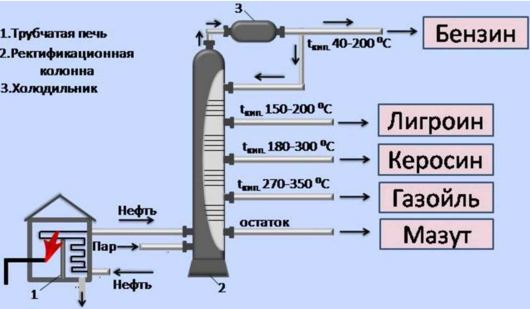
Перегонная (ректификационная) колонна
