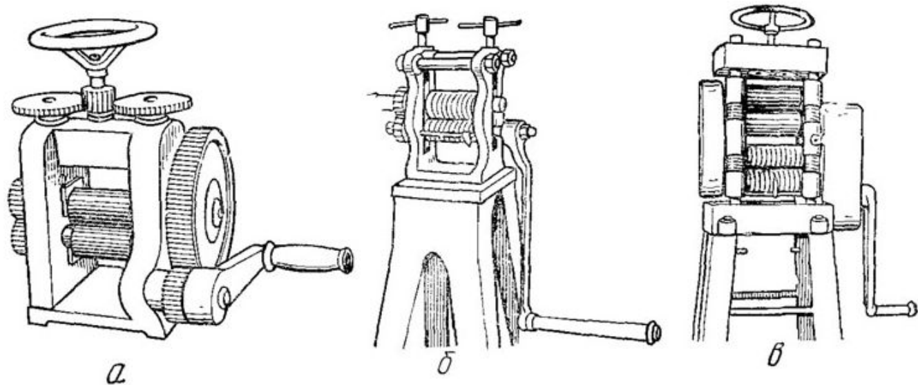
Прокатные вальцы с ручным приводом: а – плоские, б – фасонные, в – комбинированные
