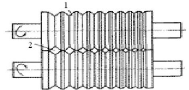
Профильные валки
