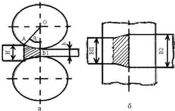
Деформация металла при прохождении его между валками
