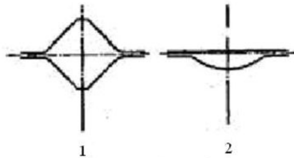
Квадратный и сегментный калибр
