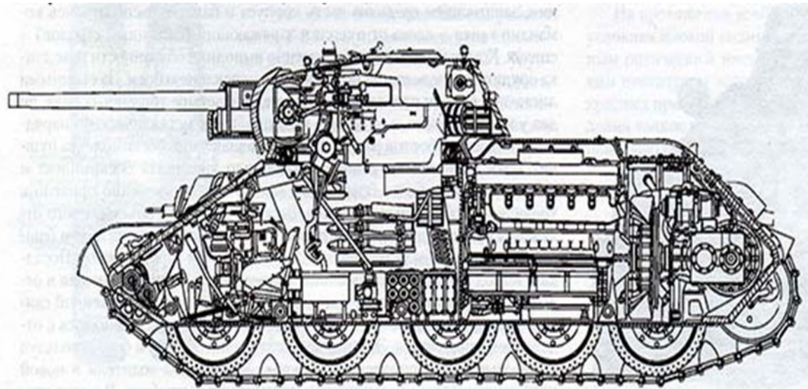
Продольный разрез танка Т-34-76 обр. 1941 г.
