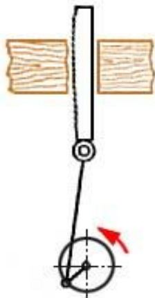
Лесопильная рама
