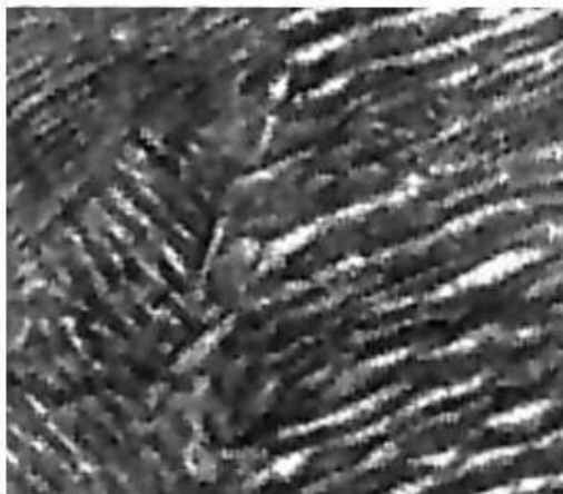
Троостит закалки
