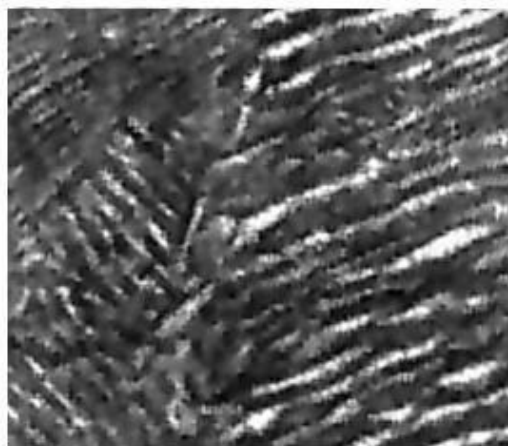
Троостит закалки
