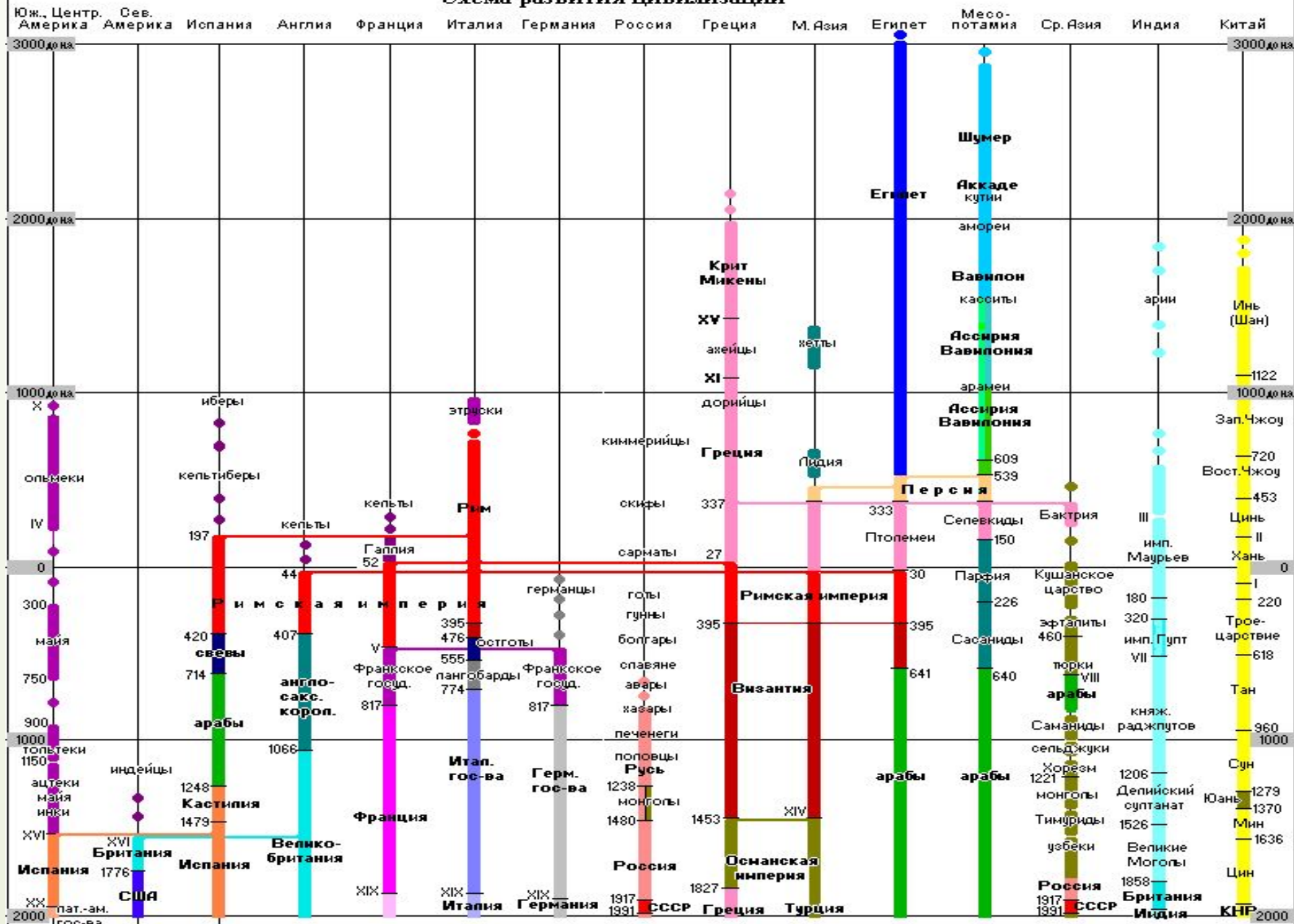
GIF версия 0.3
