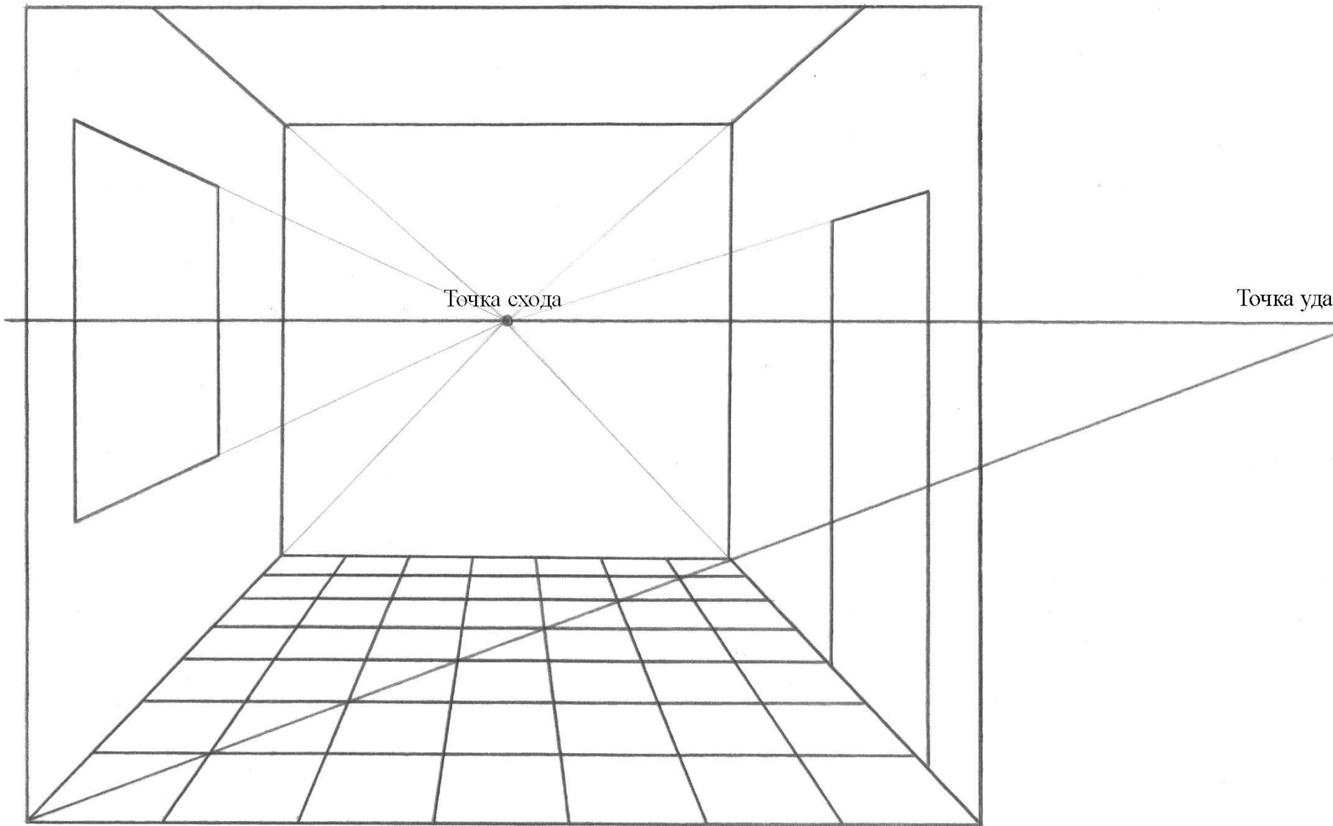
Изображение перспективного сокращения квадратов паркета
