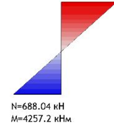
Расчетные напряжения max=3.57 МПа min=-3.08 МПа
