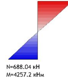
Напряжения в сечении max=3.67 МПа min=-3.11 МПа
