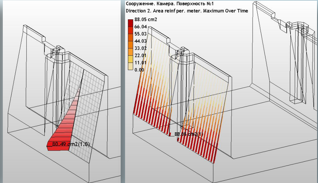
Интенсивность армирования
