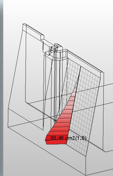
Интенсивность армирования
