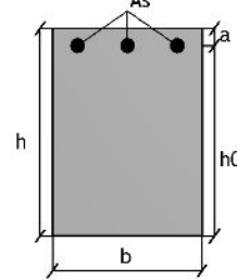
Эскиз сечения A_s
