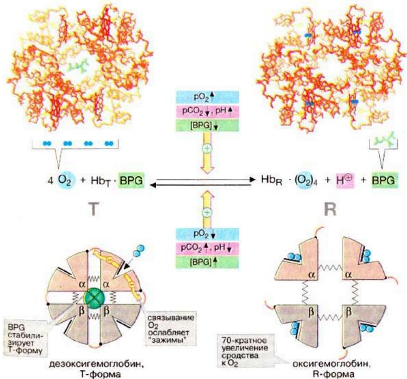
Б. Аллостерические эффекты в гемоглобине
