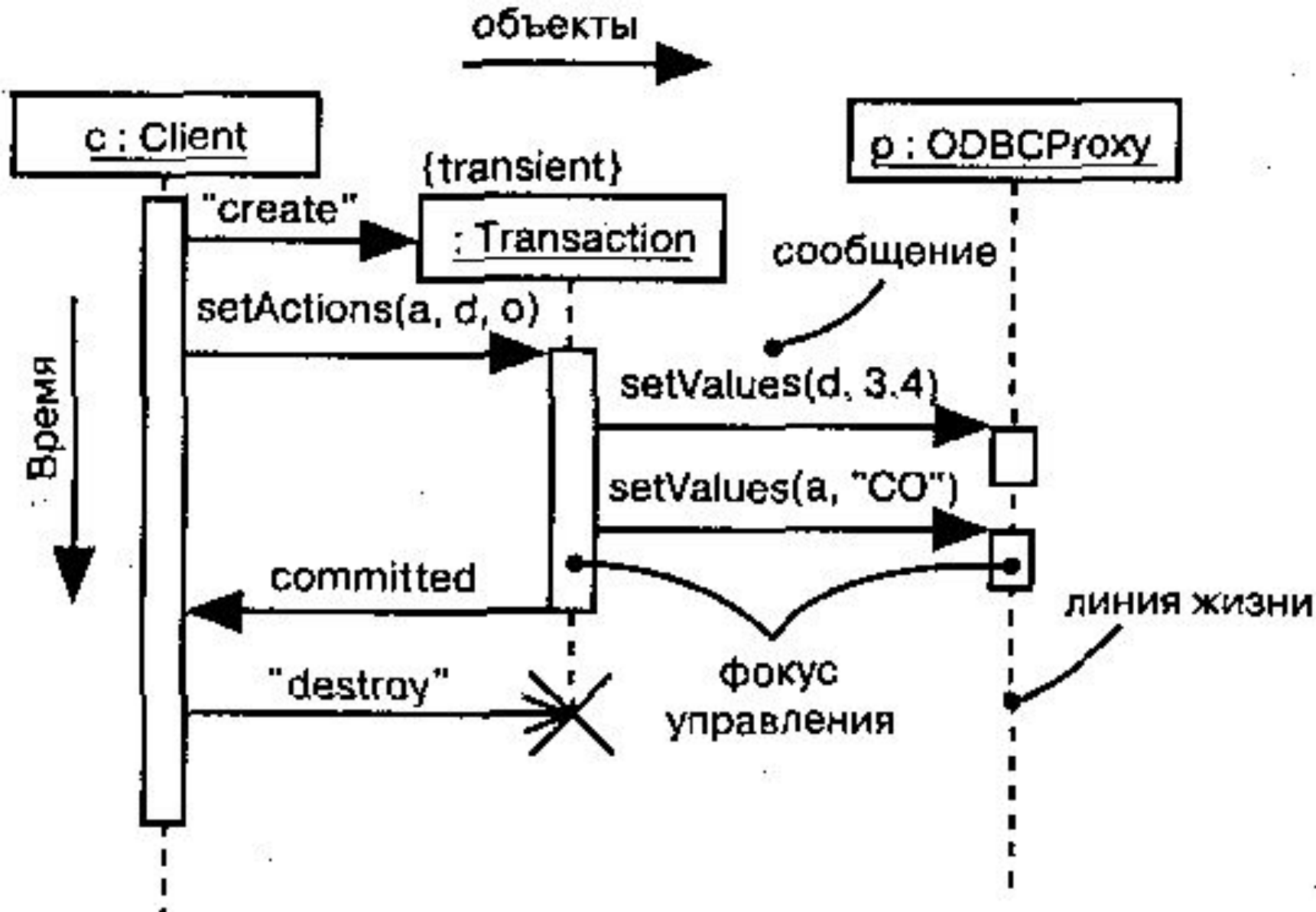
Рис. 7. Диаграмма последовательностей
