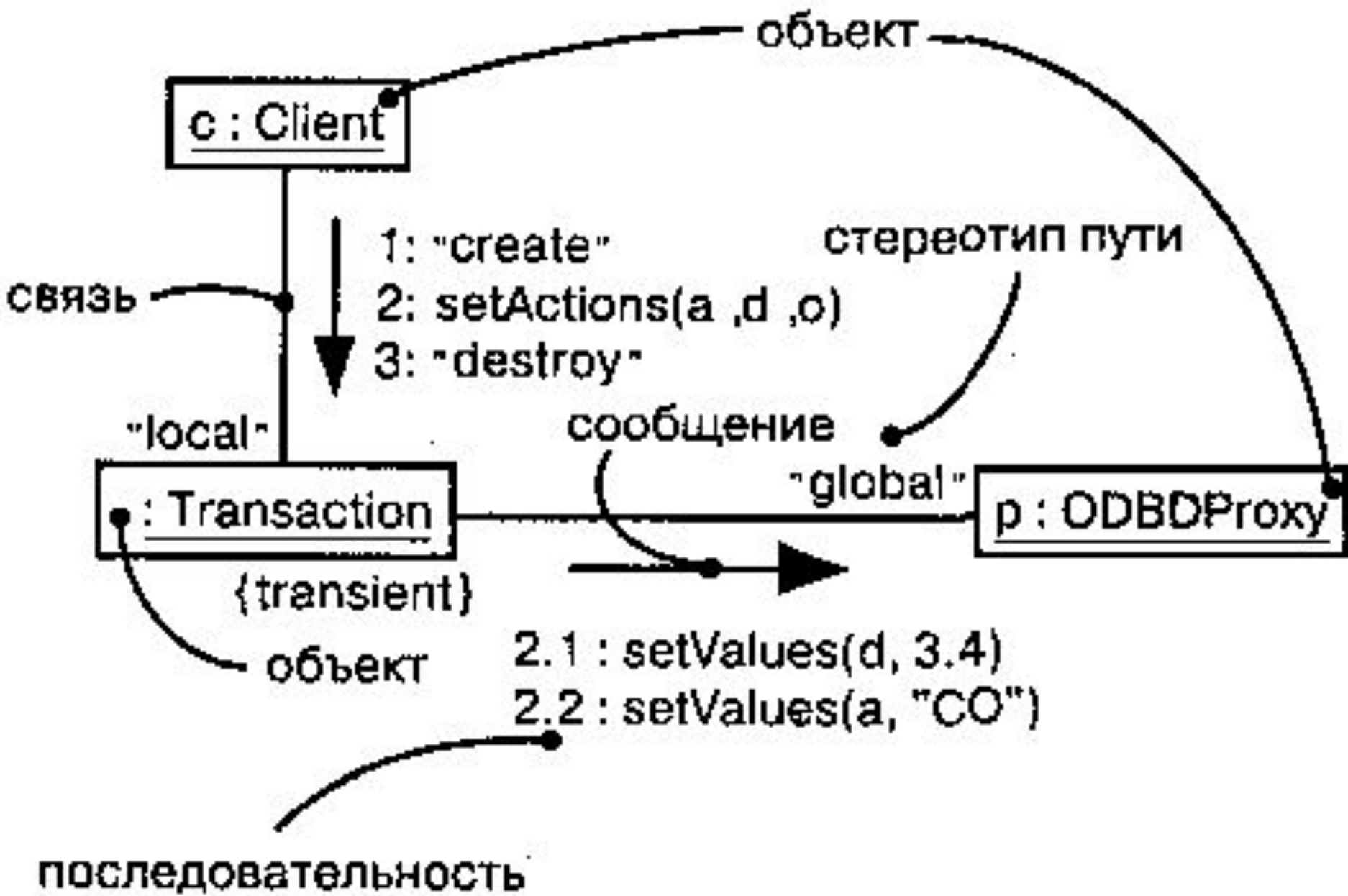
Рис.8. Диаграмма кооперации 11
