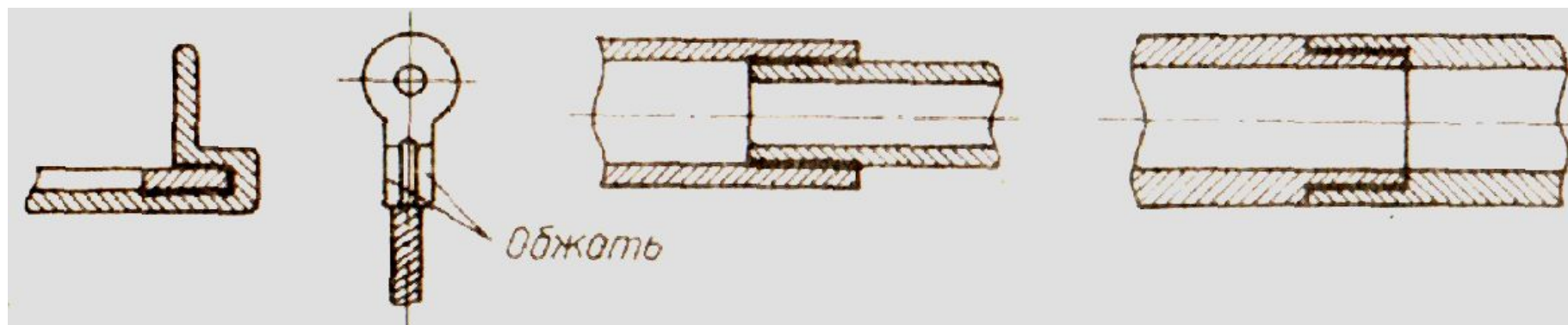
Рис. 4.10. Примеры соединения деталей с помощью замазки
