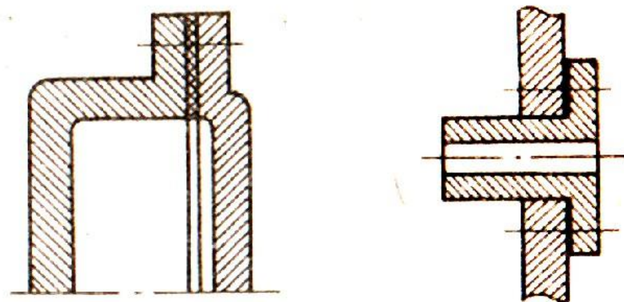
Рис. 4.12. Соединения невысыхающей замазкой
