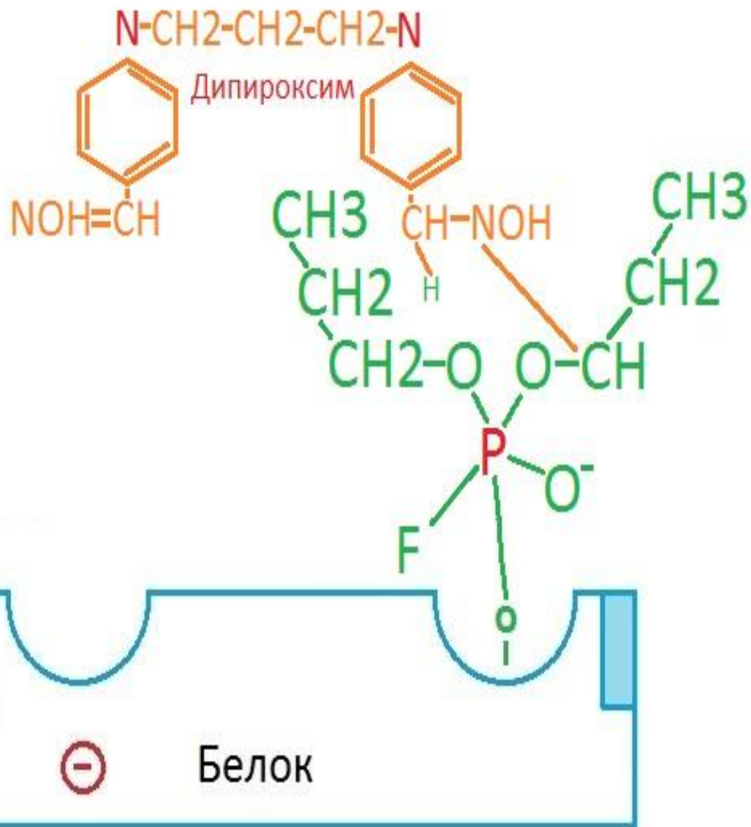
Анионный центр
