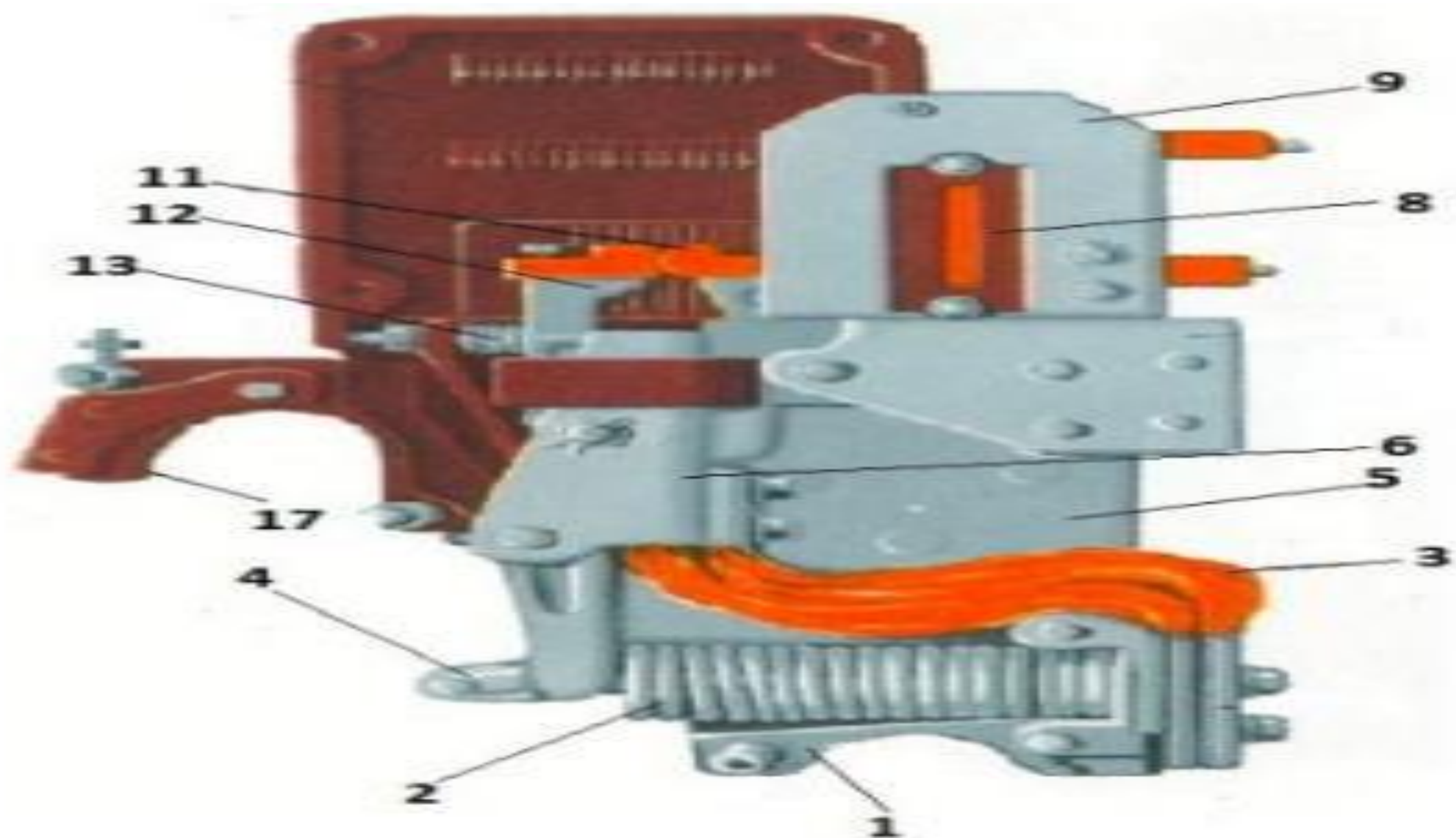
контактор с дугогашением
