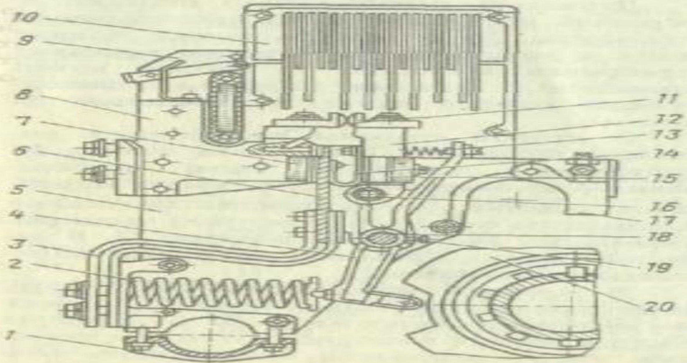
Устройство контактора с дугогашением:
