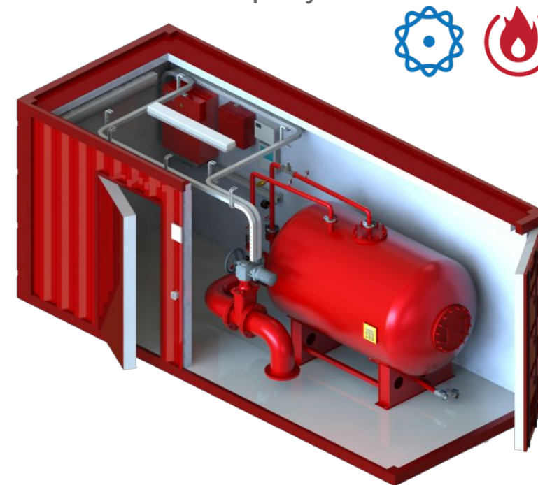
Блок Контейнер пенного пожаротушения
