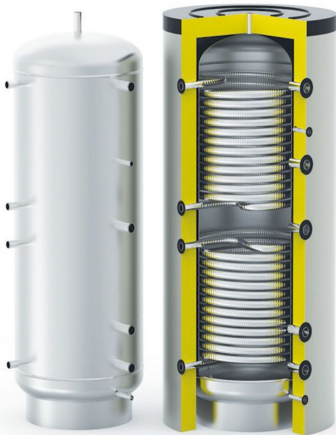
Тепловой аккумулятор
