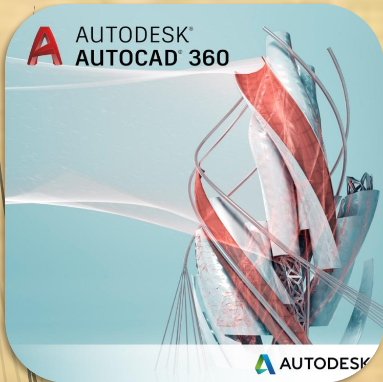
AutoCad 360
