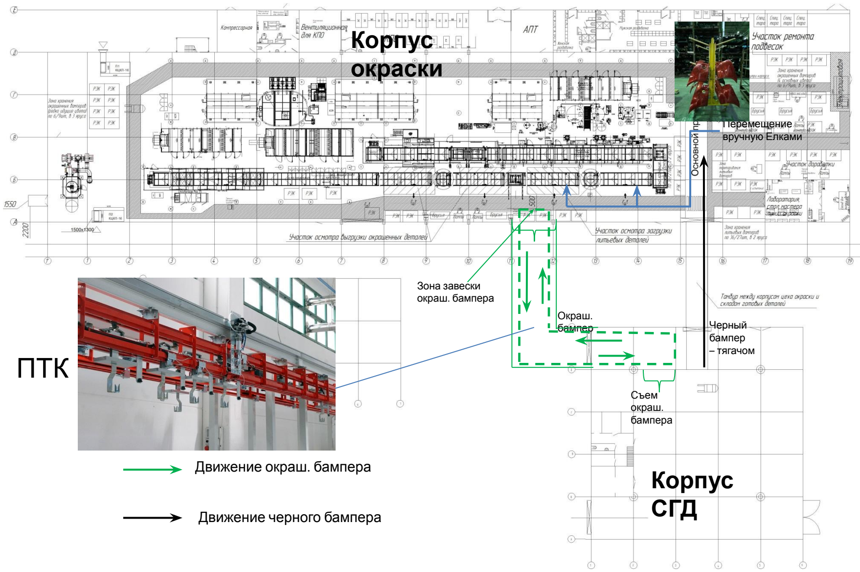
Схема движения окрашенных бамперов
