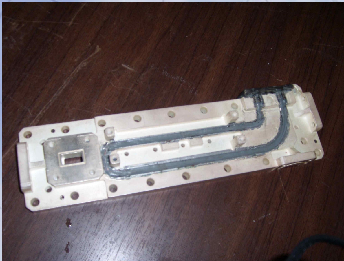
ВВУМ 3 – система охлаждения
