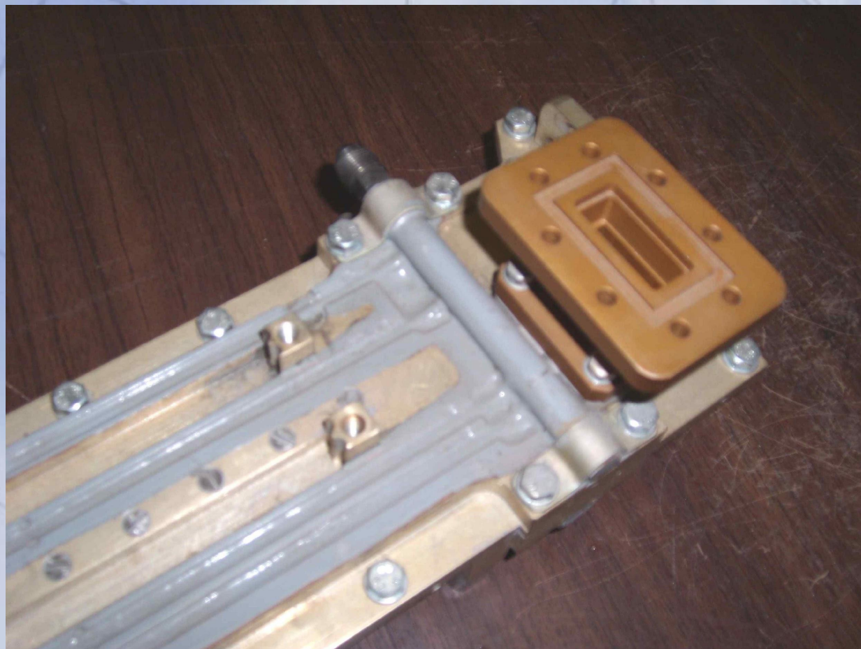
ВВУМ 2 – система охлаждения
