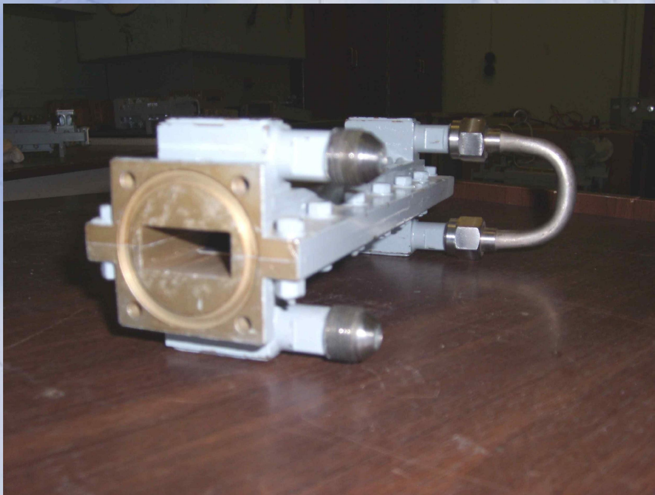
ВВУМ 1 – ферритовая нагрузка
