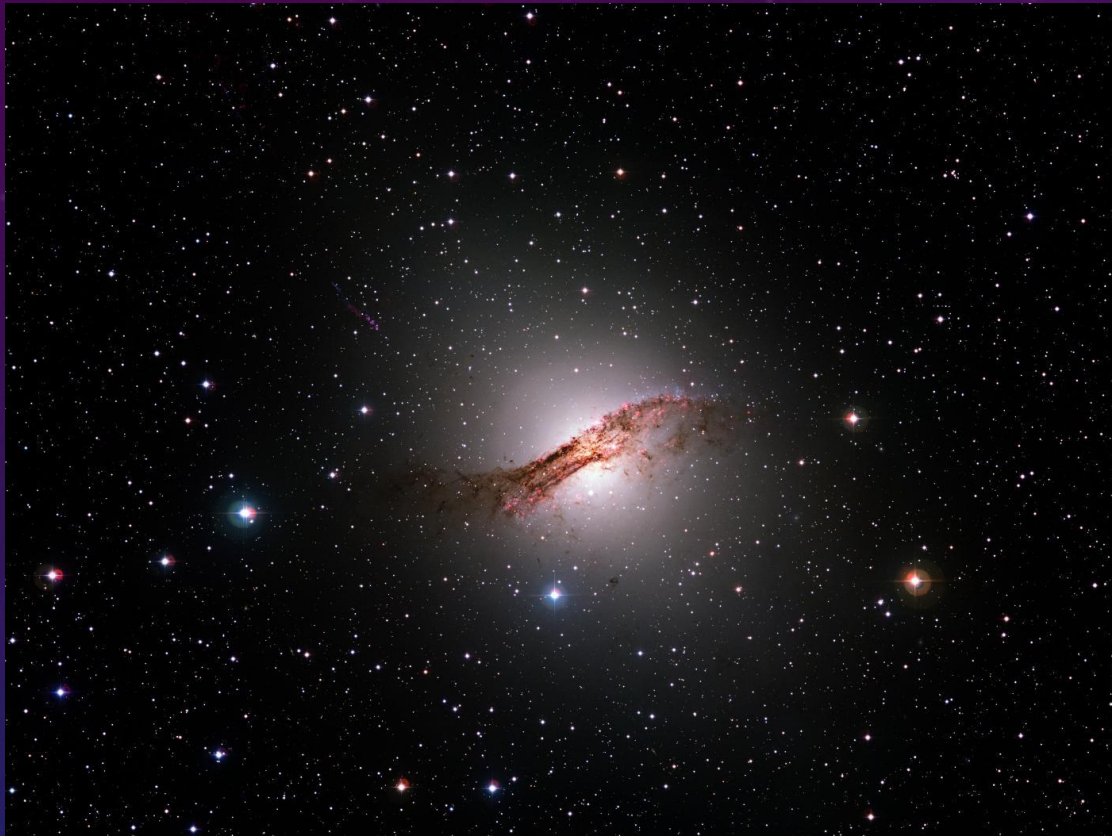
CENTAURUS A
