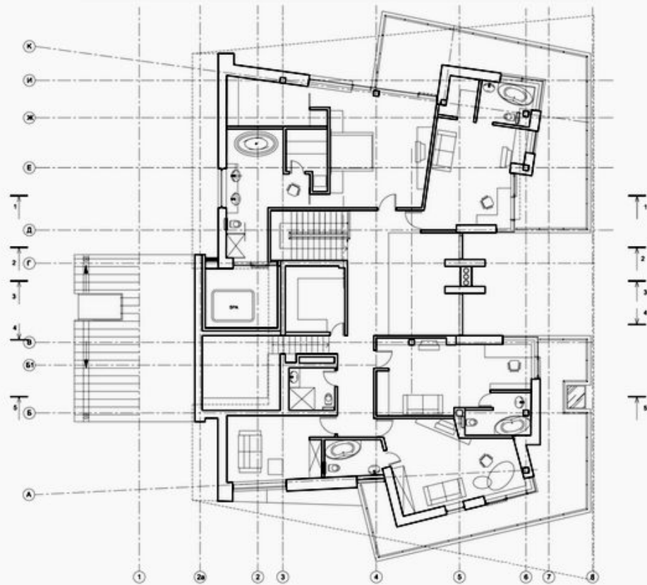
ПЛАН 2-ГО ЭТАЖА/2ND FLOOR PLAN
