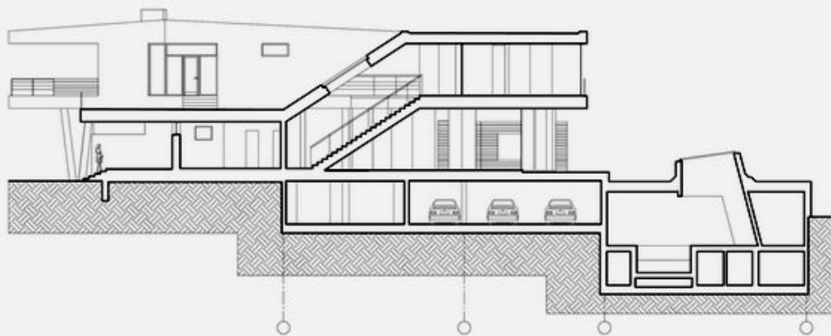
РАЗРЕЗ 1-1/SECTION 1-1
