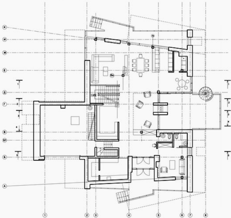
ПЛАН 1-ГО ЭТАЖА/1ST FLOOR PLAN
