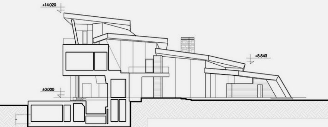
РАЗРЕЗ 1-1/SECTION 1-1
